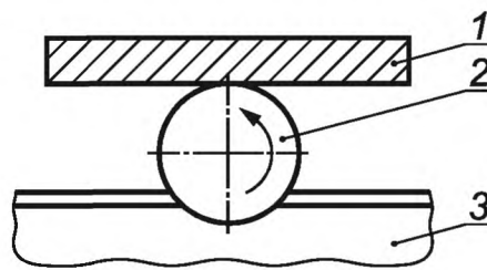
1 — образец; 2 — валик; 3 — битум
