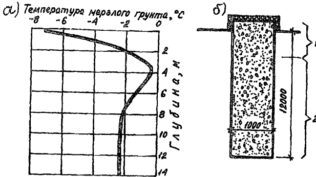
Рис.6. Температура грунта (а) и схема буронабивной свай (б): 1 - зона электропрогрева бетона, 2-зона термосного выдерживания бетона
