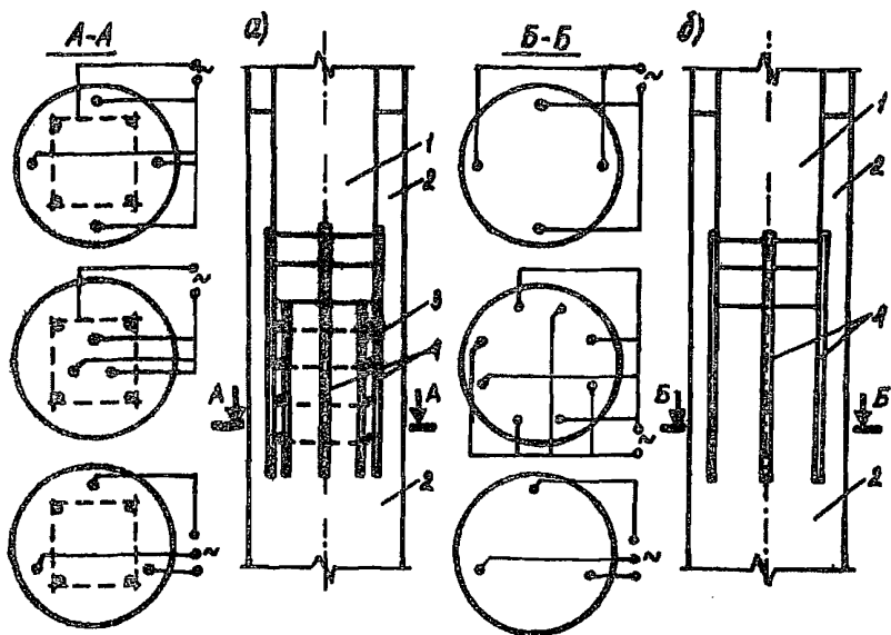
Рис. 2. Схемы размещения и подключения электродов при прогреве бетона в стьке комбинированных свай при наличии выпусков арматуры в теле сборного железобетонного элемента (а) и без выпусков (б); 1 - сборный элемент, 2 - монолитный бетон, 3 - выступающий арматурный каркас, 4 - стержневые электроды
