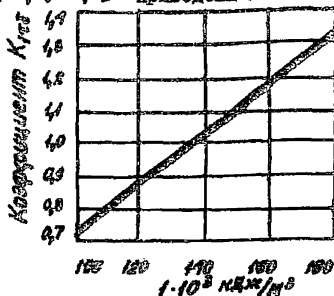
Рис.4. Значение коэффициента K_i для показателей \tau и \delta буронабивных свай, где 100-180 - суммарное тепловыделение бетона за период 28 сут твердения в нормальных условиях ( 1 \cdot 10^3 ккал/м 3 )
