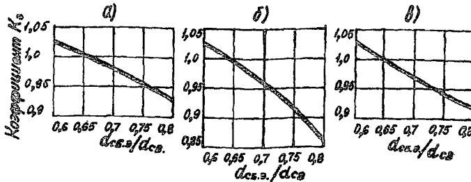
Рис.5. Значение коэффициента K_s для показателей R (а), \delta (б) и \tau (в) комбинированных свай, где 0,6-0,8 - соотношение диаметров сборного элемента и монолитной части свай ( d_{cs.o.}/d_{cs.} ). Показатели R , \delta и \tau приведены в табл.1-3
