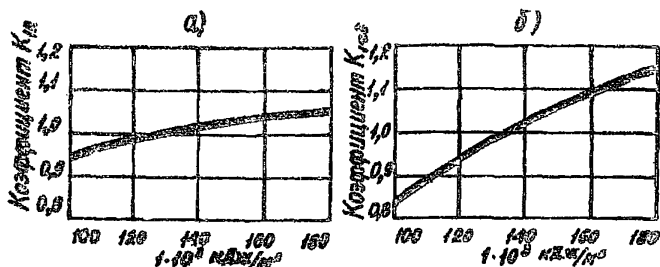
Рис.3. Значение коэффициента K_i для показателей R (а) и \delta (б) комбинированных свай, где 100-180 - суммарное тепловыделение бетона за период 28 сут твердения в нормальных условиях ( 1 \cdot 10^3 ккал/м 3 ). Показатели R , \delta , \tau приведены в табл. I-3.
