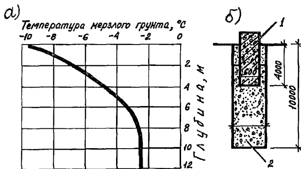
Рис.7. Температура грунта (а) и схема комбинированной сваи (б): 1-сборный железобетонный элемент, 2-монослитный бетон
