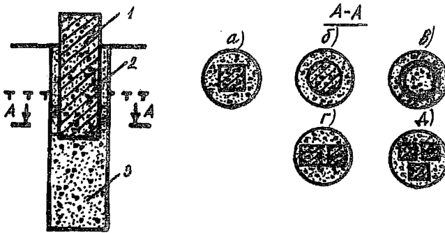
Рис. 1. Конструктивные схемы комбинированных свай (а, б, в, г, д): 1—сборный железобетонный элемент, 2—раствор, 3—монолитный бетон
