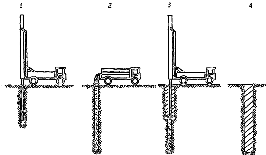
Рис.2. Технологическая схема изготовления цементогрунтовой свай по способу ИВ:
