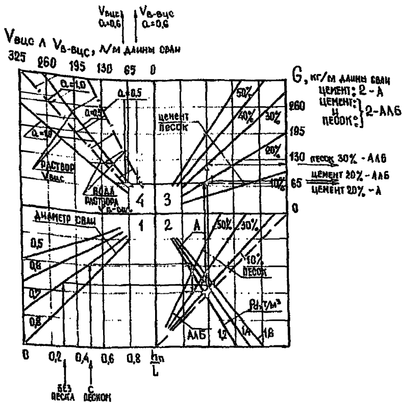
Рис. 2. Номограмма для определения параметров:
