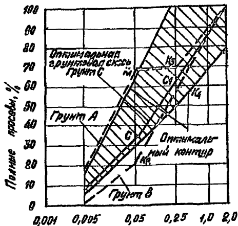
Рис. 2. Проектирование состава грунта по кривым полных просевов
