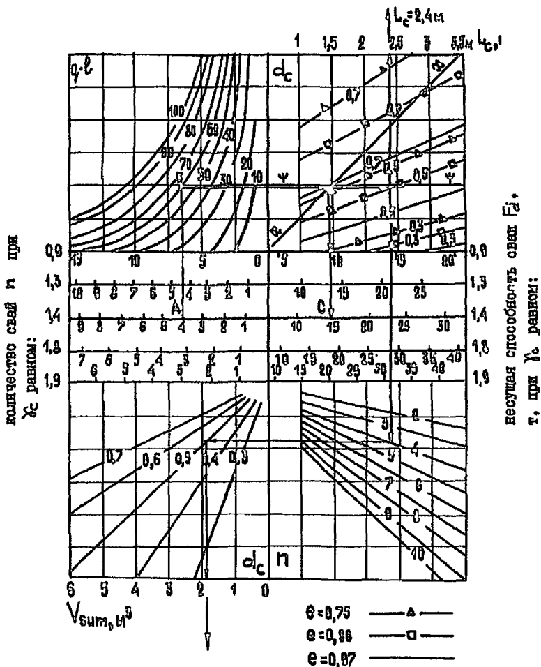
Нограмма для определения значений в зависимости от значения интенсивности равномерно распределенной нагрузки, грунтовых условий и типа зданий для свай длиной от 1 до 3,5 м на просадочных грунтах (см. табл. 3)
