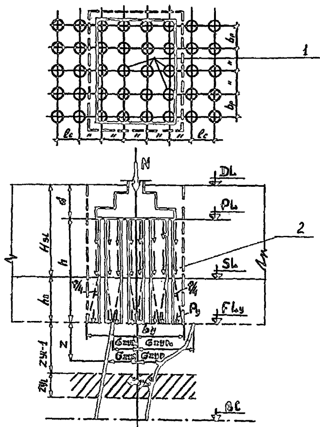
Рис.1. Схема расчета осадок основания, армированного цементогрунтовыми сваями
