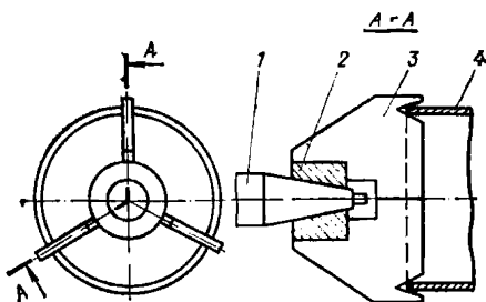
Рис. 28. Переходное приспособление для крепления пневмобойника к забиваемой трубе
