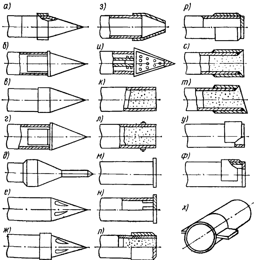
Рис. 1. Наконечники для прокладки труб способом прокола
