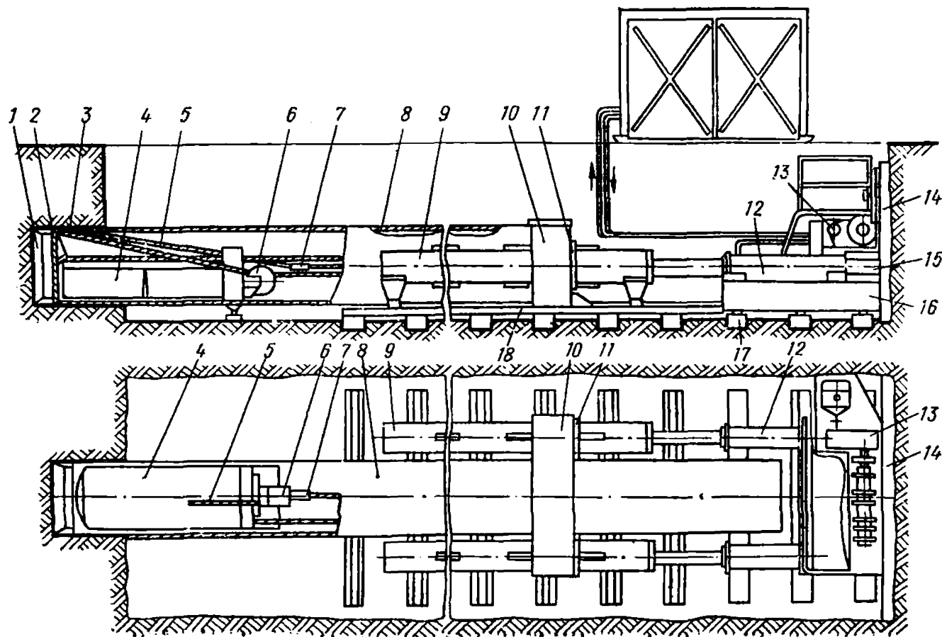
Рис. 25. Установка СКБ Главмос- стройка
