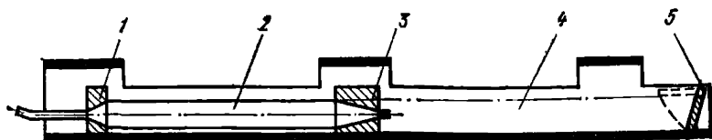
Рис. 29. Самоходная капсула для очистки кожухов от грунта
