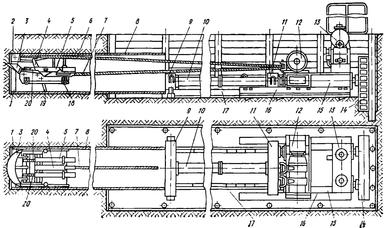
Рис. 26. Установка ПУ-2
