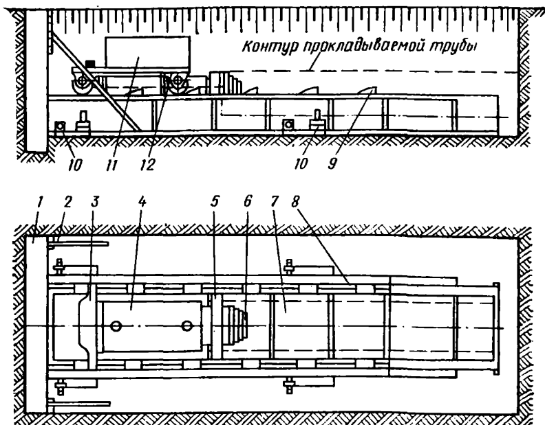
Рис. 5. Установка Главмостроя для прокладки труб способом прокола
