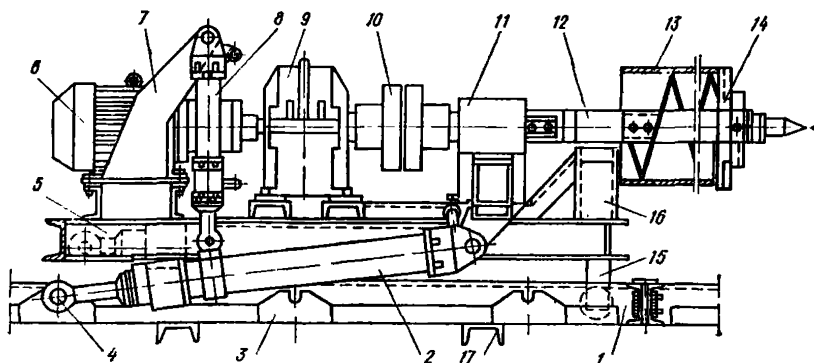
Рис. 38. Буровая машина ГБГ-600
