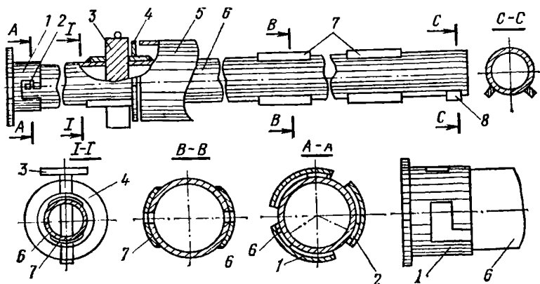
Рис. 3. Штанга-шомпол
