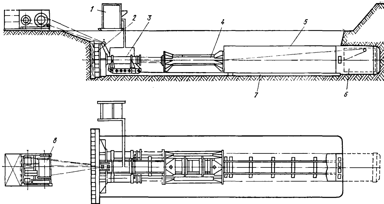
Рис. 27. Установка для бестраншейной прокладки труб У-12/60
