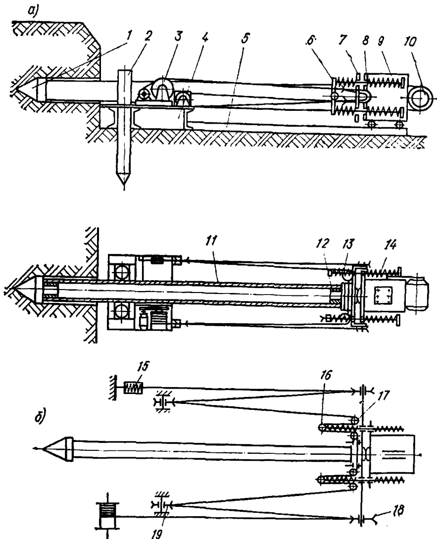
Рис. 21. Установка УВВГП-400
