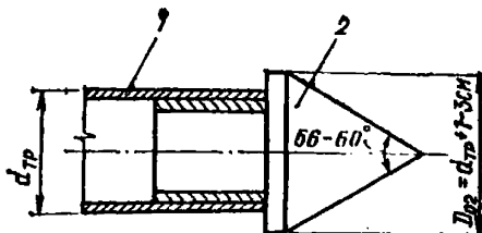
Рис. 15. Инвентарный оголовок
