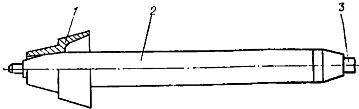
Рис. 17. Переходная втулка
