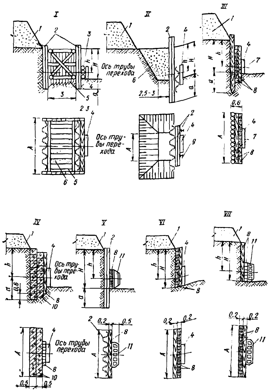
Рис. 23. Типовые упорные стенки для прокладки кожухов методами прокалывания и продавливания
