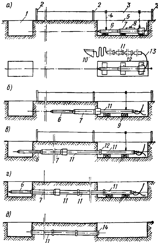
Рис. 20. Схема производства работ по прокладке асбестоцементных труб
