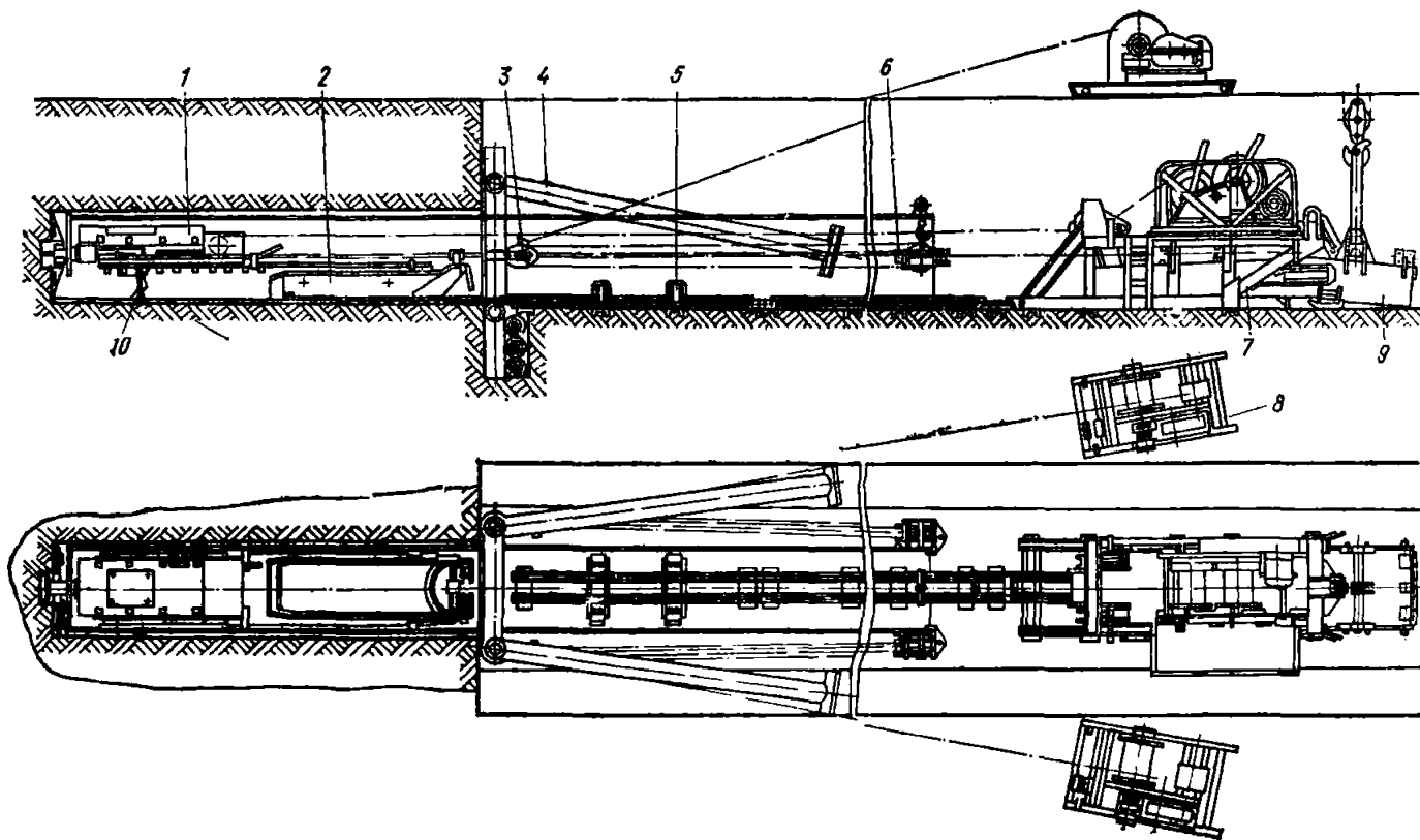
Рис. 36. Машина для бес-траншейной прокладки труб ПМ-800-1400
