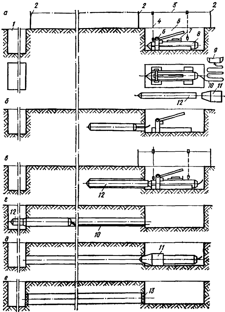
Рис. 9. Схема производства работ при пробивке скважин пневмопробойником
