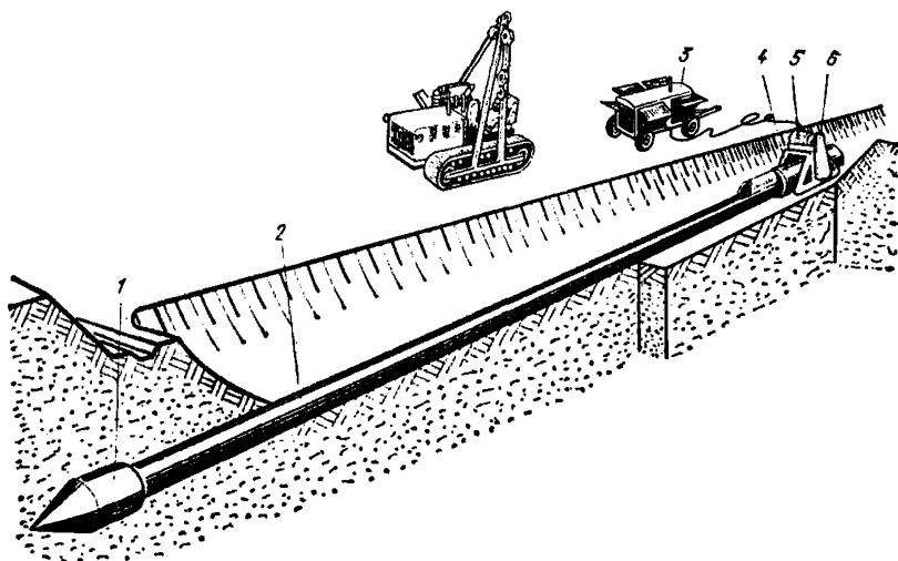
Рис. 31. Схема бестраншейной прокладки трубопровода установкой УВГ-51
