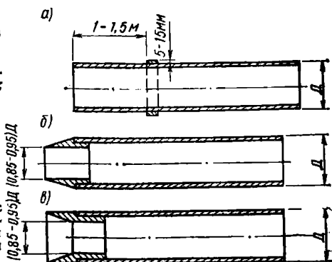
Рис. 30. Варианты конструктивного оформления переднего торца трубы
