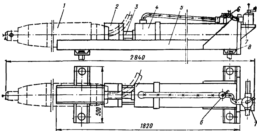
Рис. 11. Схема стартового устройства для пневмопробойника СО-134 (ПР-400)
