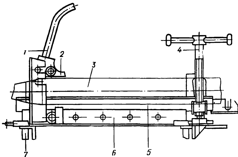
Рис. 10. Схема стартового устройства для пневмобойников ИП-4603 и ИП-4605
