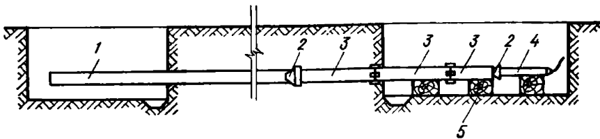
Рис. 18. Схема производства работ по замене трубопроводов
