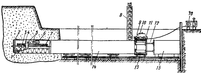
Рис. 37. Установка ГБ-1621
