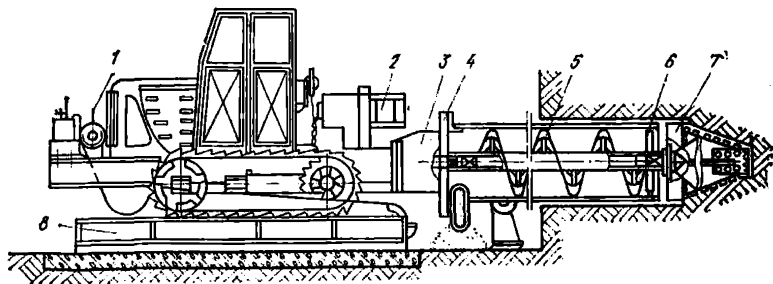
Рис. 35. Установка УГБ на базе трактора
