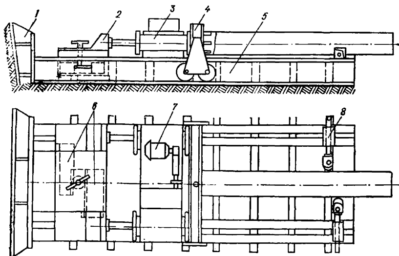
Рис. 4. Схема грунтопрокалывающей установки ГПУ-600
