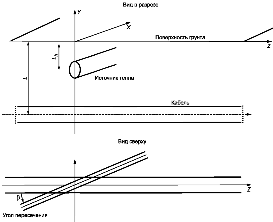
Рисунок 1 — Пример расположения источника тепла, пересекающего рассматриваемый кабель
