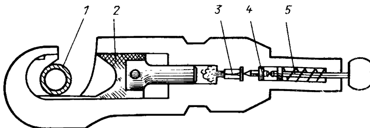
Рис. 7. Резка стальной трубы прессом ПРТ:
