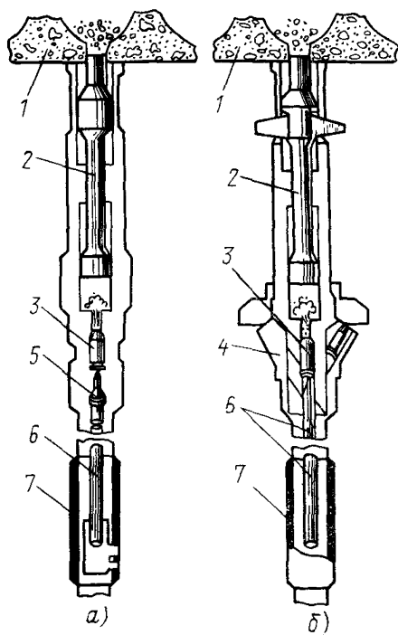
Рис. 5. Выполнение отверстий ударными колонками УК-6 (а) и УКМ (б):
