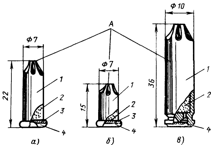
Рис. 8. Монтажные патроны для порохового инструмента шифров Д (а), К (б) и МПУ (в)
