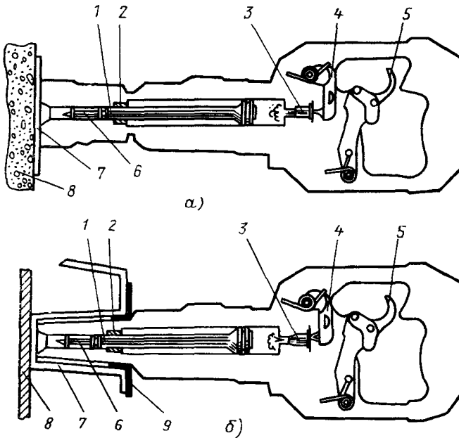
Рис. 1. Крепление дюбелями с применением пистолетов ПЦ84 (а) и ПЦ84С (б):
