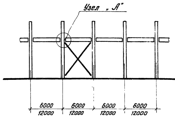
Схема опирания стальных подкрановых балок на колонны в связевой панели
