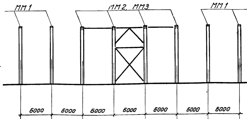
По крайним рядам при шаге 6 м
