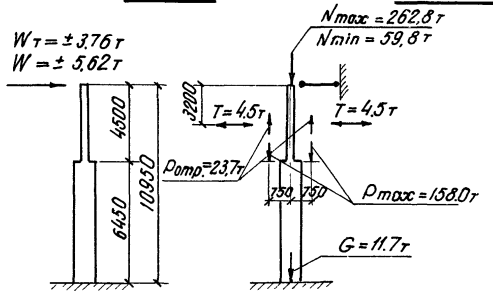
Расчетная схема
