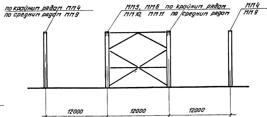
по крайним и средним рядам при шаге стропильных конструкций 12 м Схема установки закладных элементов в колоннах по серии КЭ-01-56. при применении стальных ферм
