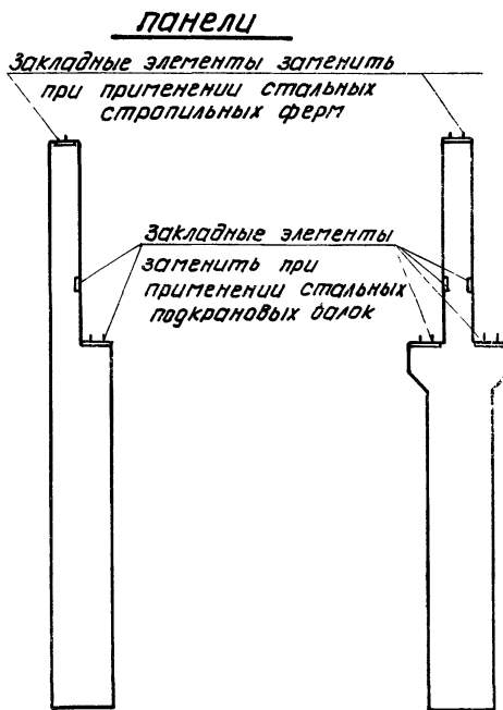
Схема опирания стальных подкрановых балок на колонны в связевой панели
