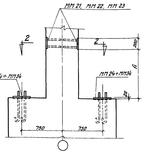
Колонна по среднему ряду
