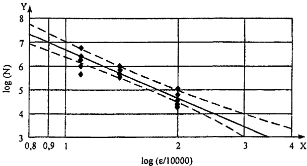
Рисунок 6 — Пример графика усталости асфальтобетонного образца
