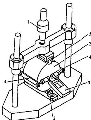
1 – нагружающее устройство; 2 – образец; 3 – тензомер; 4 – деформационные полосы; 5 – нагружающие полосы Рисунок 2 – Нагружающая установка
