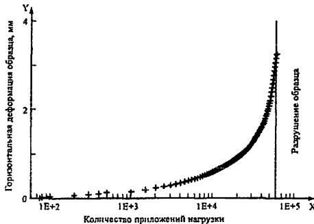
Рисунок 7— Определение срока разрушения образца
