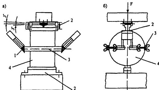
1 – деформационная полоса; 2 – нагружающая полоса 3 – тензомер; 4 – образец
