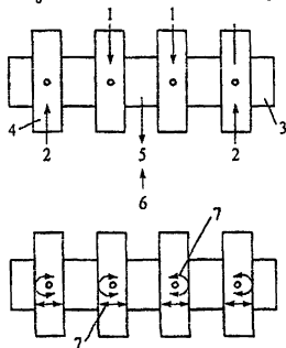
1 – прикладываемая нагрузка; 2 – направление сопротивления прикладываемой нагрузки; 3 – образец; 4 – зажим образца; 5 – направление прогиба; 6 – направление возвращения образца в исходную позицию; 7 – свободная передача и вращение зажимов Рисунок 1 — Основные принципы испытания образцов по четырехточечной схеме
