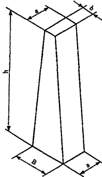
Рисунок 4 – Трапециевидная форма асфальтобетонного образца
