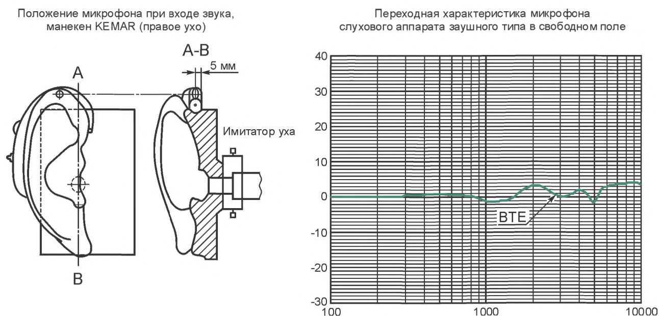
Рисунок А.1 — Положение микрофона и соответствующая переходная характеристика микрофона слухового аппарата заушного типа в свободном поле
