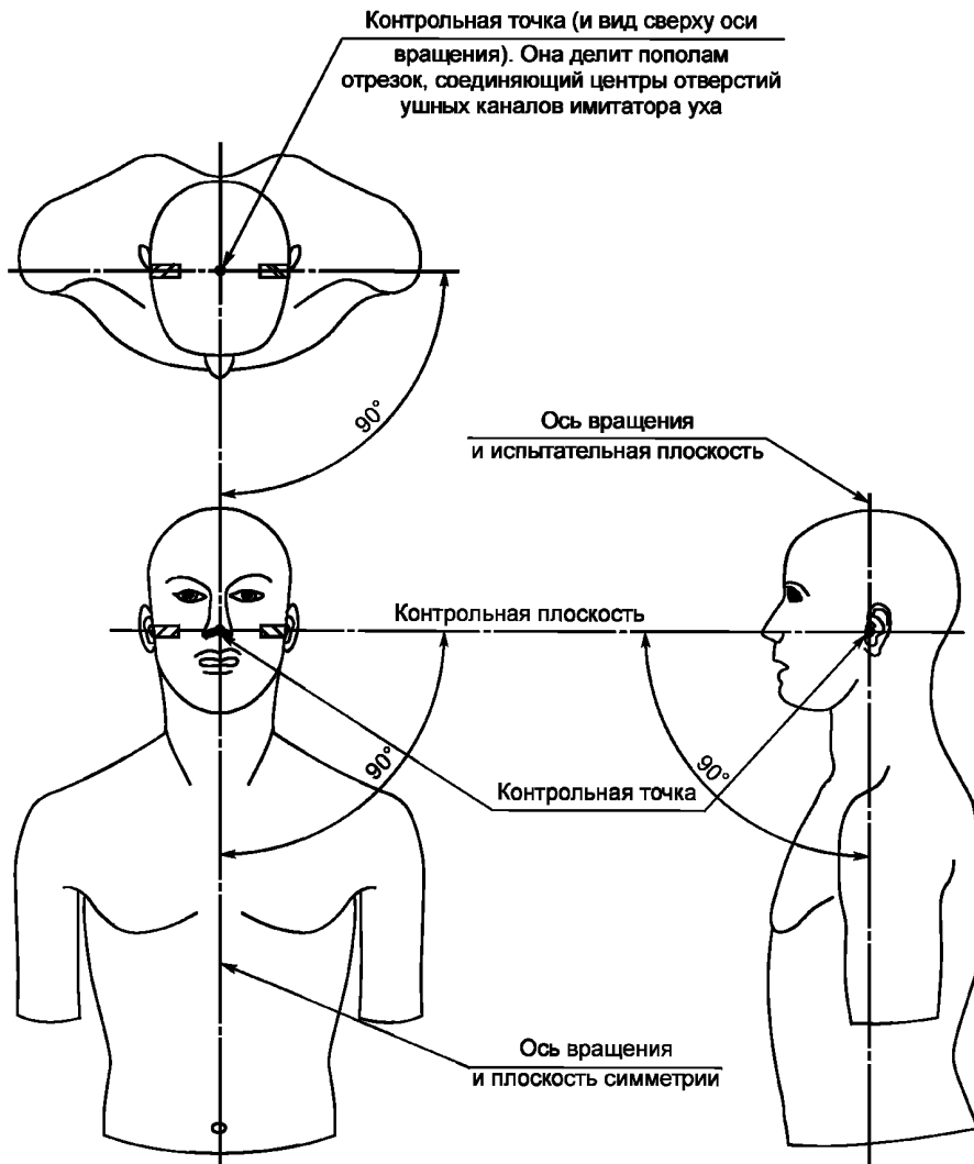
Рисунок С.1 — Геометрические характеристики манекена
