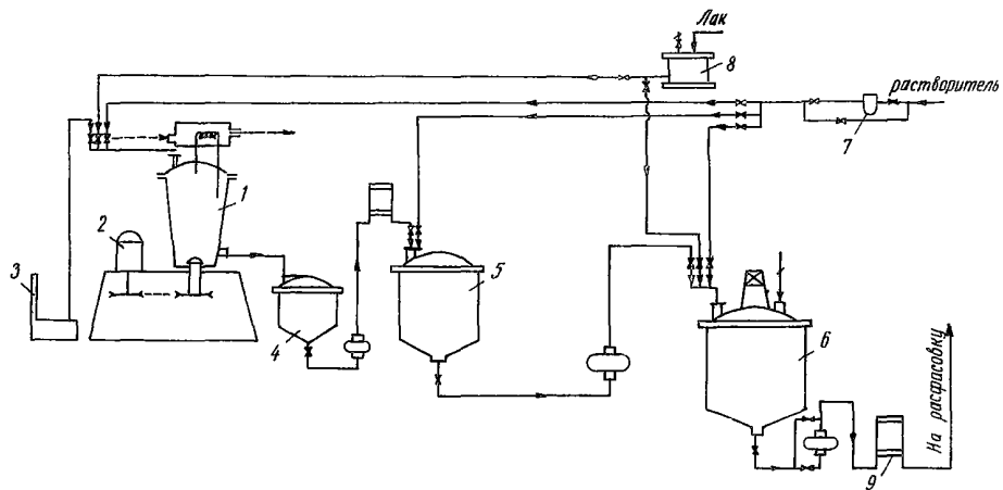
Рис.2. Технологическая схема производства ХПБМ
