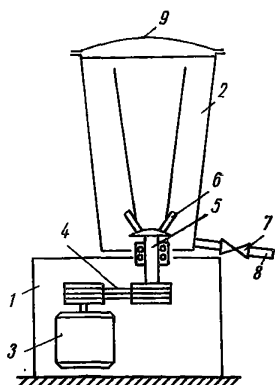
Рис. I. Схема диспергатора ВД-75 1 - рама; 2 - емкость; 3 - электродвигатель; 4 - клиноременная передача; 5 - вал мешалки; 6 - мешалка пропеллерная; 7 - сливной кран; 8 - сливной патрубок; 9 - крышка емкости
