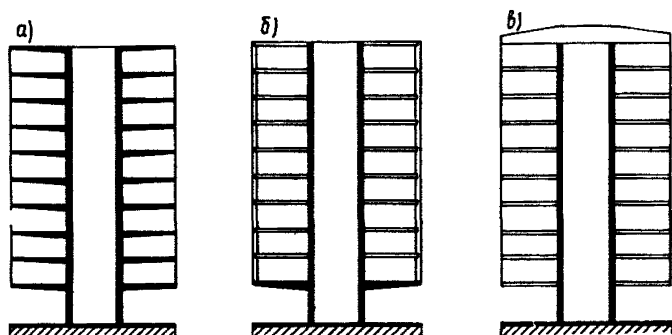
Рис. 5. Конструктивные решения здания с незастроенным первым этажом
