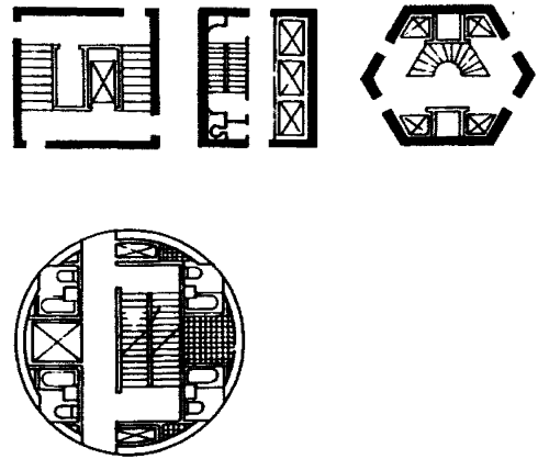
Рис. 2. Примеры планировочных решений монолитных ядер жесткости
