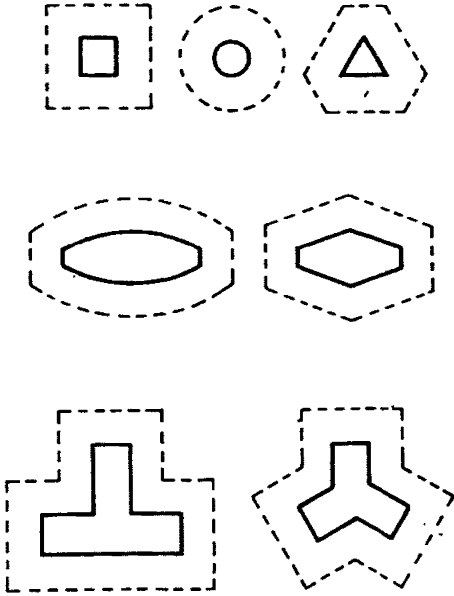
Рис. 1. Варианты планов монолитных стволов и зданий
