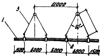
Рис. 4. Схема строповки звена труб. 1 - звено трубы ( l=20m ); 2 - П-820 3 - строп 2х ветевой
