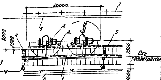
Рис. 3. План укладки стальных труб в траншею
