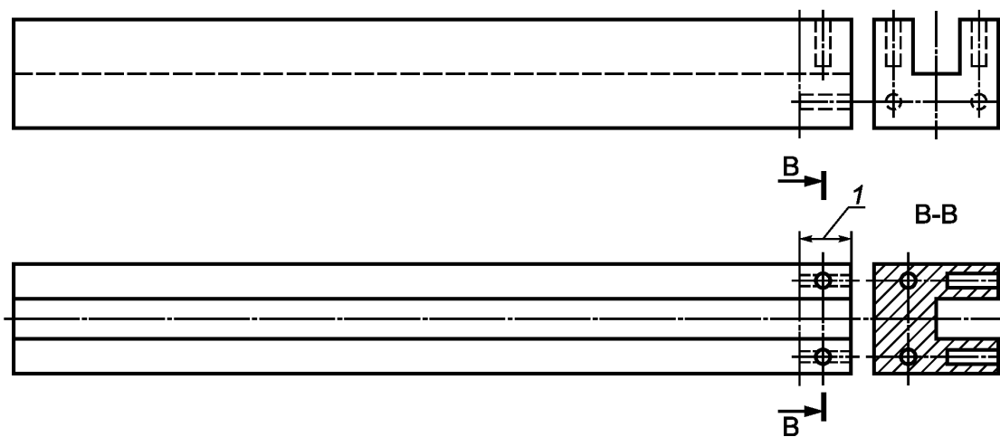
Рисунок 2 — Места отбора проб от подовых блоков, спрессованных с пазом
