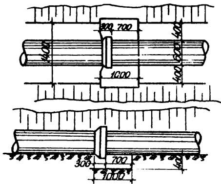
Рис. 3. Приемок для заделки отыка
