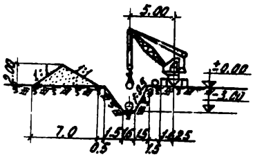
Разрез по б-б
