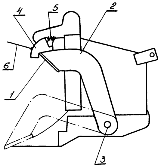
Рис. 2 Струга для зачистки дна траншеи экскаватором.
