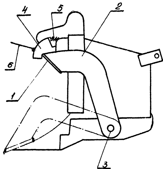
Рис.4 Струг для зачистки дна траншеи экскаватором 1-Нож струга; 2-упорные штанги; 3-цапфа; 4-замк.-защелка; 5-пружина; 6-тросик.
