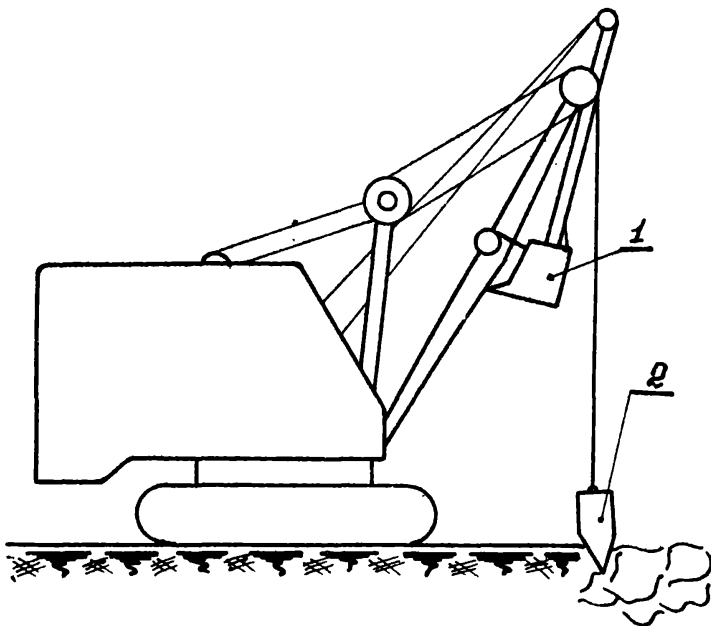
рис. 3 Схема установки стенного оборудования на экскаваторе Э-65В
