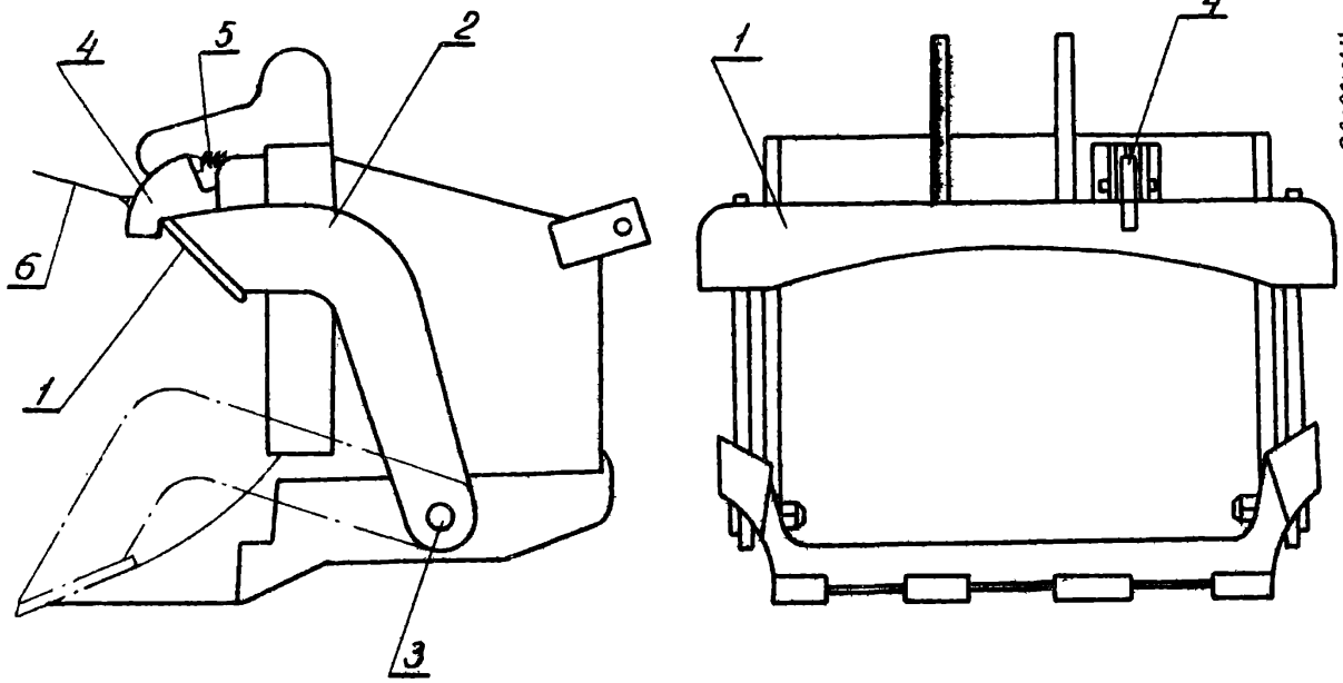
Рис. 4 Струв для зачистки дна траншеи экскаватором. 1-нож струва; 2-ударные штанги; 3-цангра; 4-замок-защелка; 5-пружина; 6-тросик
