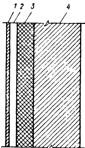
Рис. 2. Конструкция стены с вентилируемой прослойкой
