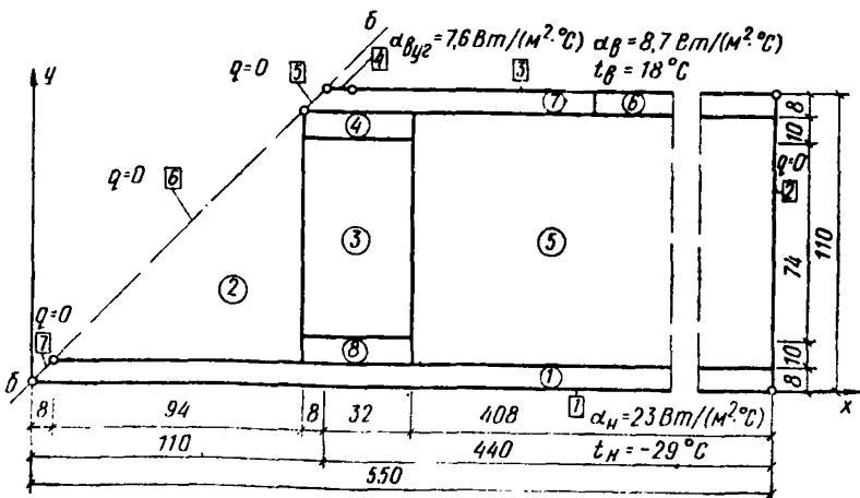
Рис. 20. Чертеж исследуемой области
