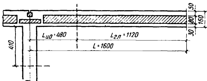
Рис. 15. Схематический чертеж фрагмента неоднородной ограждающей конструкции
