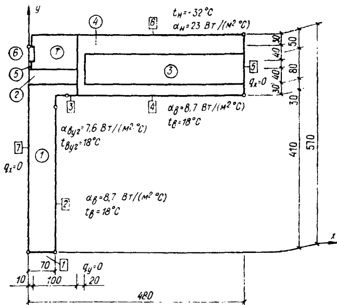
Рис. 16. Чертеж исследуемой области
