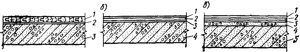
Рис. 6. Конструкции полов к примерам 1 и 2
