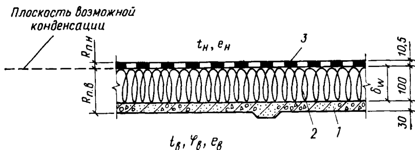
Рис. 9. Сечение неветилируемого покрытия коровника для расчета требуемого сопротивления паропрооницанию
