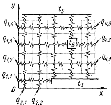
Рис. 5. Эквивалентная электрическая цепь стационарного поля
