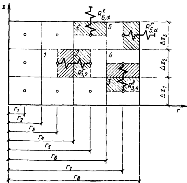
Рис. 7. Схема фрагмента эквивалентной цепи для осесимметричного температурного поля
