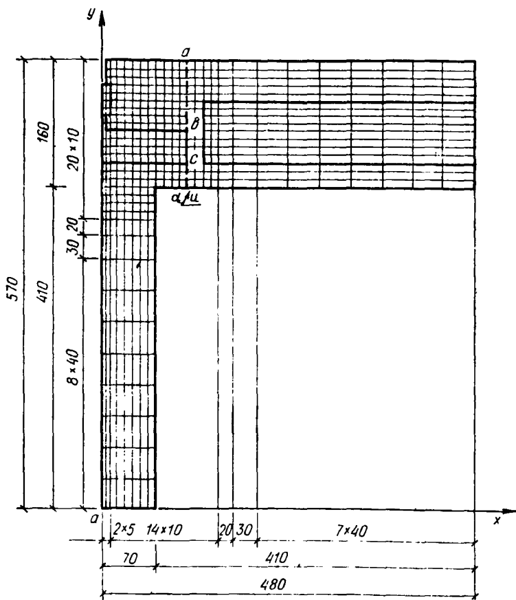
Рис. 17. Чертеж исследуемой области, расчлененной на элементарные блоки
