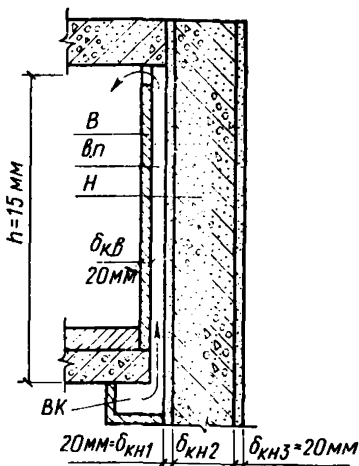
Рис. 8. Схема стены с внутренней вентилируемой прослойкой
