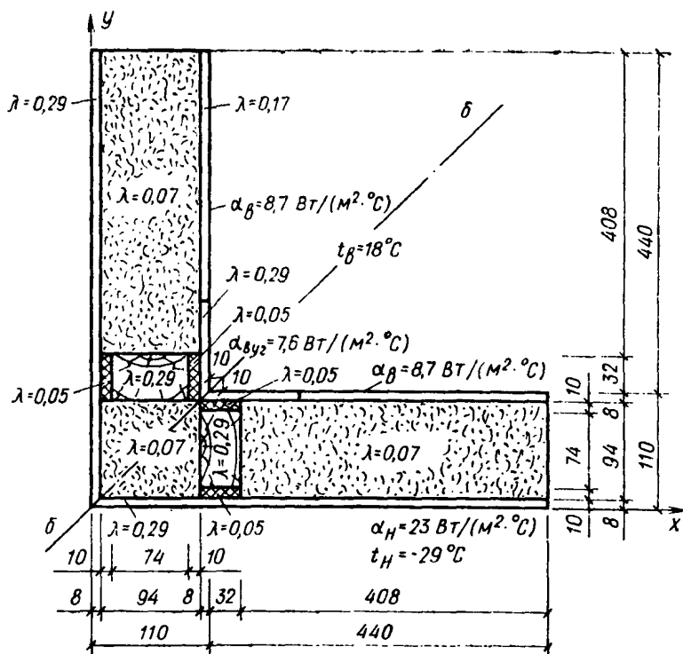
Рис. 19. Схематический чертеж углового наружного стыка
