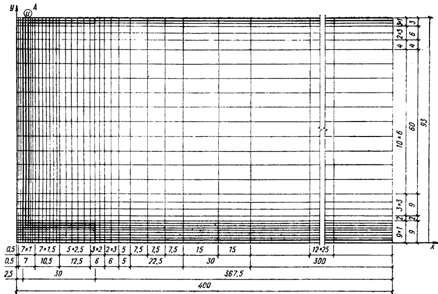
Рис. 13. Чертеж исследуемой области, расчлененной на элементарные блоки
