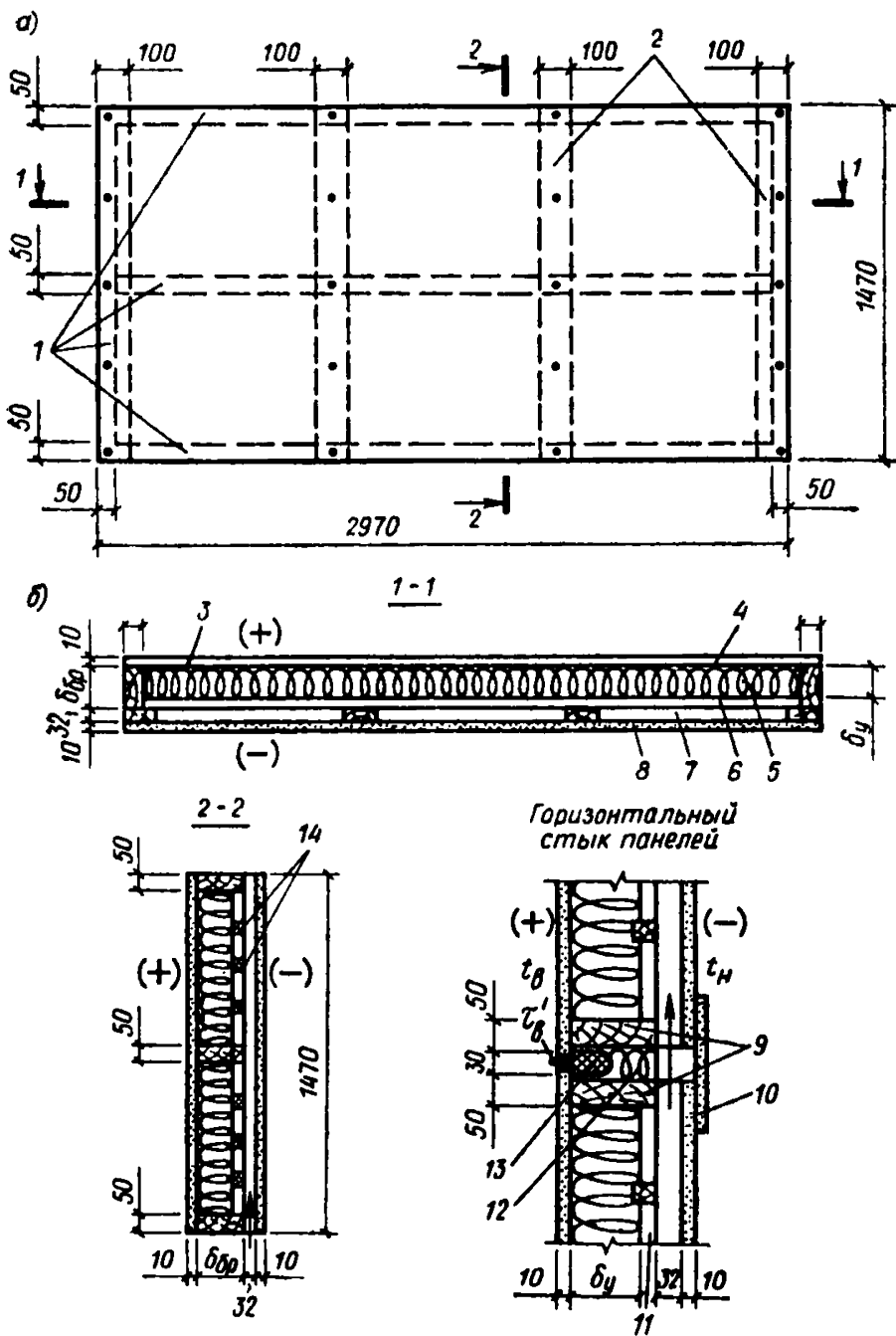
Рис. 5. Вентилируемая стенная панель с деревянным каркасом а — панель в плане: 1 — бруски каркаса; 2 — деревянные планки 100×32 мм; б — сечения 1-1, 2-2 и горизонтальный стык панелей: 3 — внутренняя асбестоцементная обшивка; 4 — пленка полиэтиленовая; 5 — плиты минераловатные, 6 — планка прижимная; 7 — вентиляруемая воздушная прослонка; 8 — наружная асбестоцементная обшивка; 9 — бруски каркаса; 10 — нащельник из асбестоцементного листа; 11 — переменный размер; 12 — минеральная вата; 13 — гернит; 14 — прижимная планка
