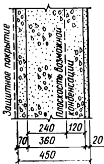
Рис. 7. Конструкция панели наружной стены промышленного здания
