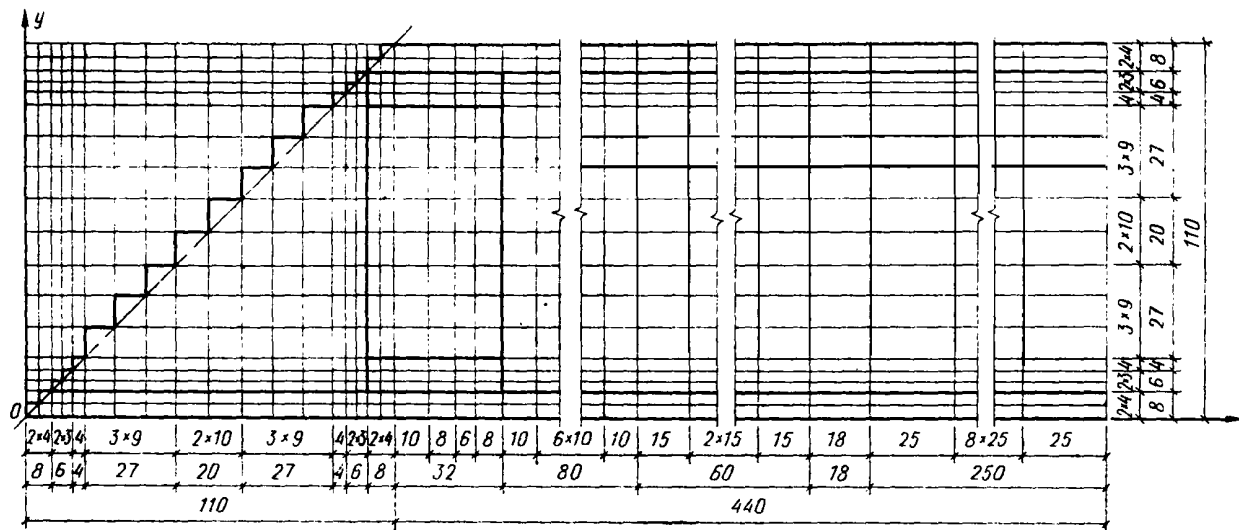
Рис. 21. Чертеж исследуемой области, расчлененной на элементарные блоки
