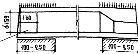
Деталь заделки торцов панелей
