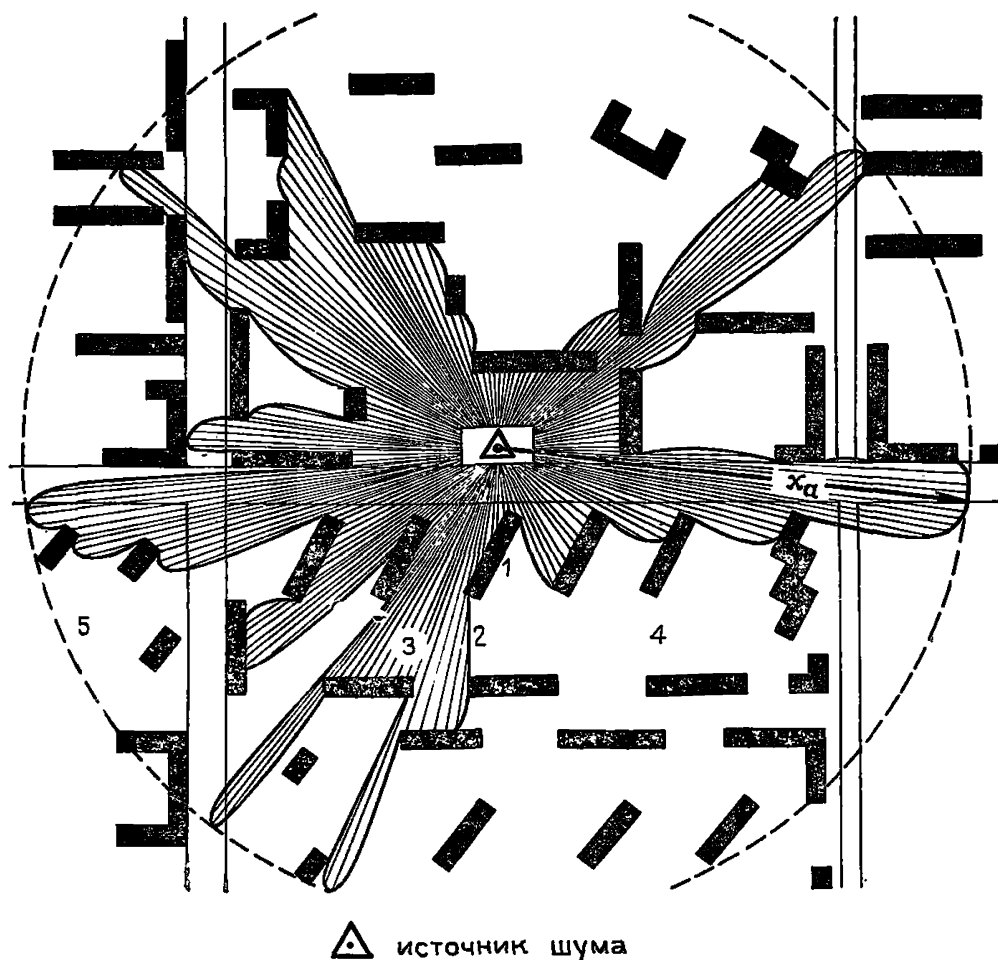
Рис. 40. Пример построения границ шумленности от точечного источника
