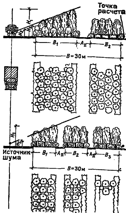
Рис. 35. Расчетная схема для определения эффективности снижения шума точечного источника боковыми частями экрана
