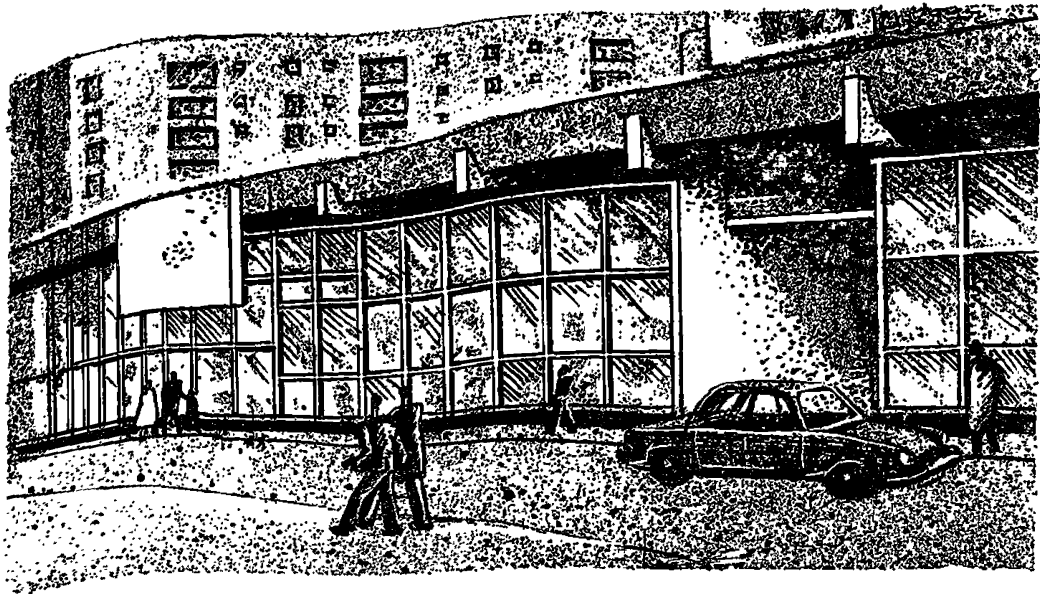
Рис. 17. Защита жилого района от шума со стороны городской улицы магазином-экраном и со стороны железной дороги — экранирующей стенкой
