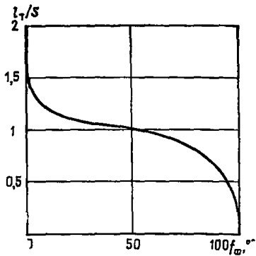
Рис. 45. График для определения времени действия фонового уровня звука f_\phi как функции отношения длины треугольника видимости источника l_T , м, к среднему интервалу между окнами S , м
