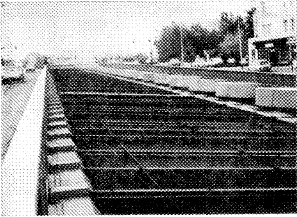
Рис. 16. Шумозащитное перекрытие из легких металлических конструкций над авто- страдой, расположенной в выемке (длина 800 м, глубина выемки 4,5 м, эффектив- ность 13 дБА, Франция)
