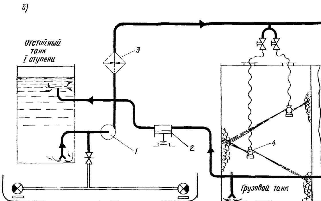
Рис. 2. Типовая схема мойки грузовых танков по замкнутому циклу: а — с двухступенчатым отстоем промывочной жидкости; б — с одноступенчатым отстоем промывочной жидкости. 1 — моечный насос; 2 — зачистной насос; 3 — подогреватель моещей воды; 4 — моечная машинка
