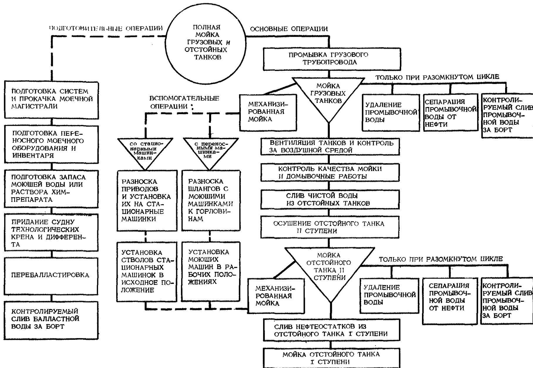
Рис. 6. Схема типового технологического процесса полной водной мойки танков
