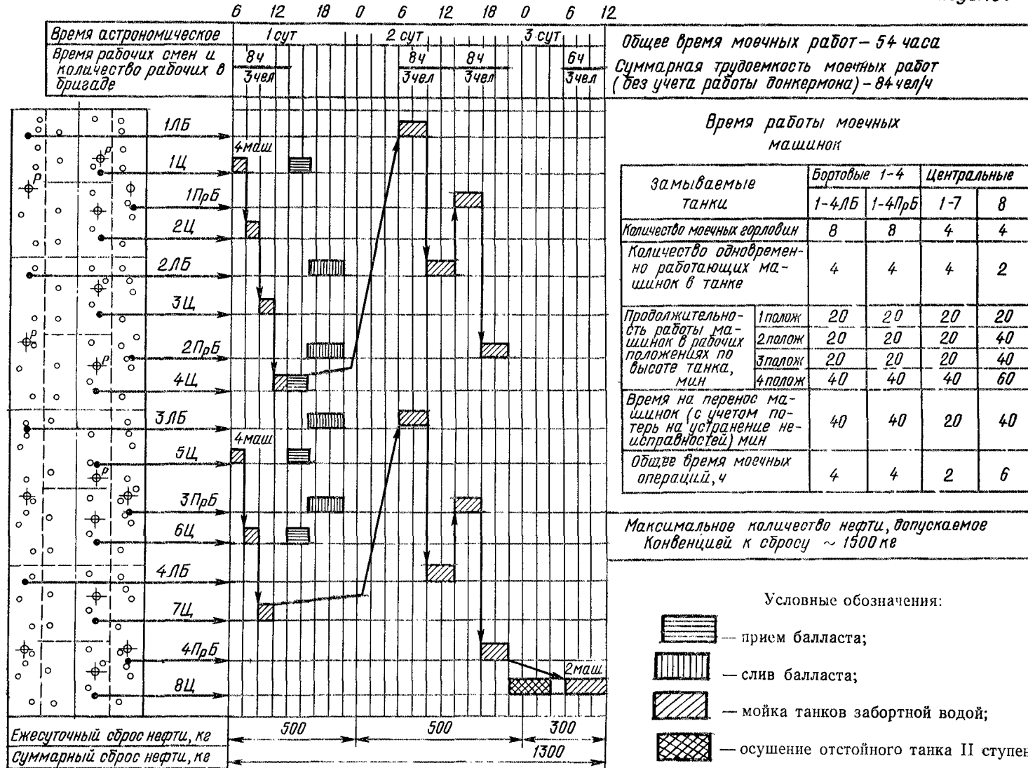
Типовой технологический график мойки грузовых танков под балластный переход
