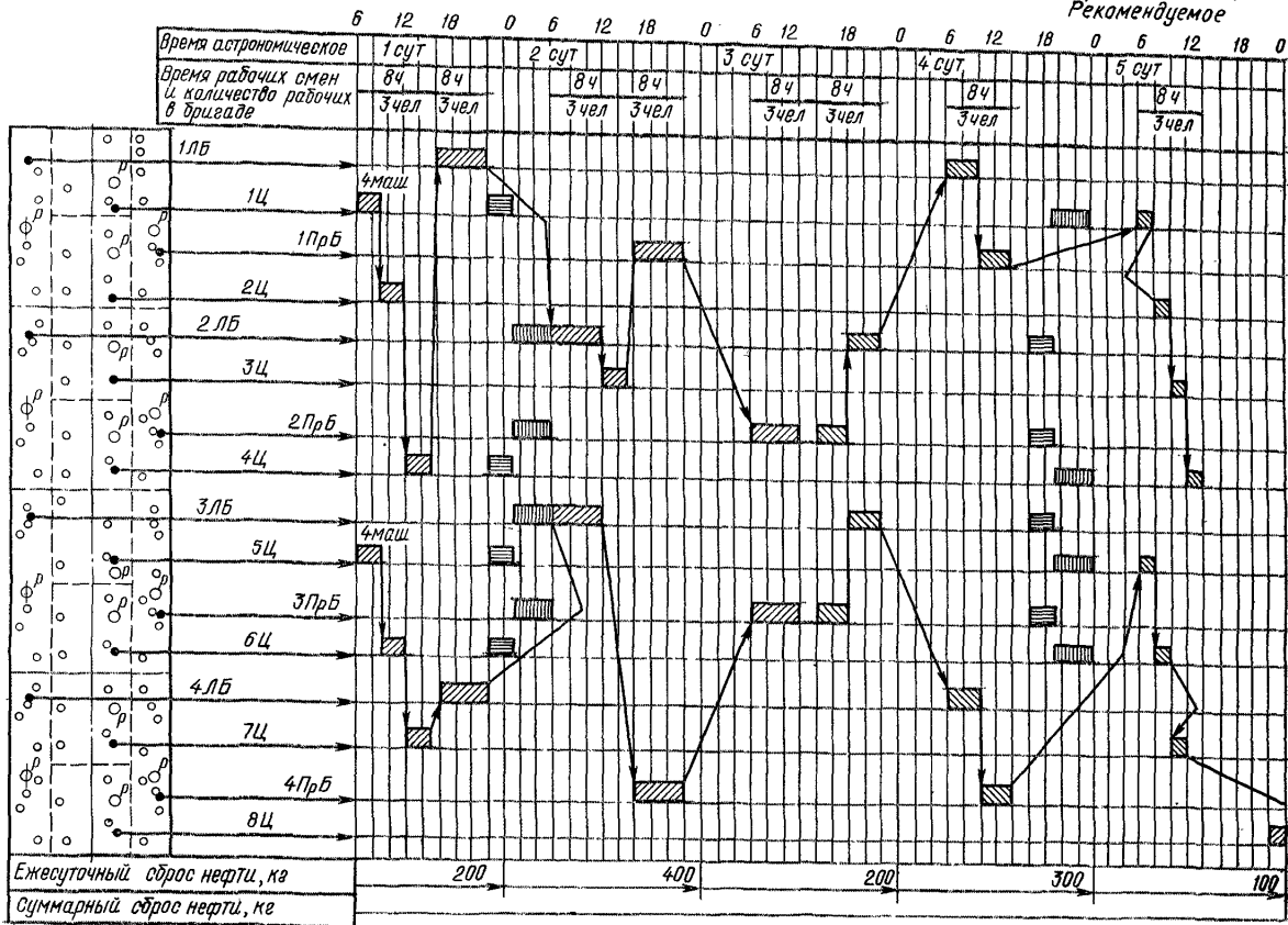
Типовой технологический график мойки танков для осмотров, профилактического удаления остатков под ремонт и смену вида груза
