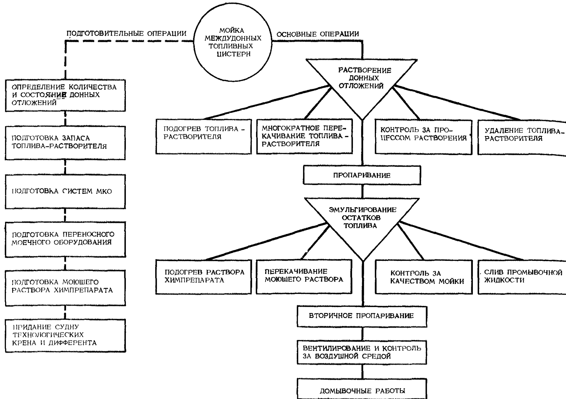
Рис. 8. Схема типового технологического процесса предремонтной мойки междудонных топливных цистерн из-под тяжелых сортов топлива
