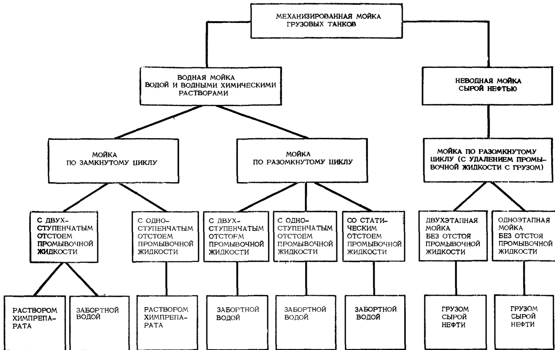
Рис. 1. Схема классификации мойки грузовых танков по способу выполнения
