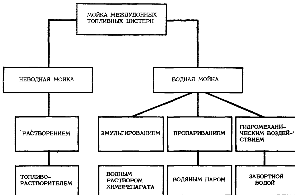
Рис. 7. Схема классификации мойки междудонных топливных цистерн по способу выполнения
