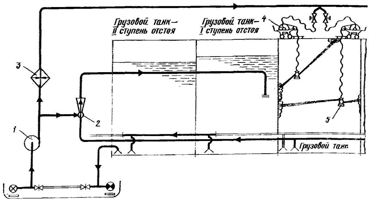
Рис. 4. Типовая схема мойки грузовых танков по разомкнутому циклу с двухступенчатым отстоем в грузовых танках при использовании эжектора в качестве зачистного средства: 1 — моечный насос (используется грузовой); 2 — зачистной эжектор; 3 — подогреватель моющей воды; 4 — шланговая лебедка; 5 — моечная машинка
