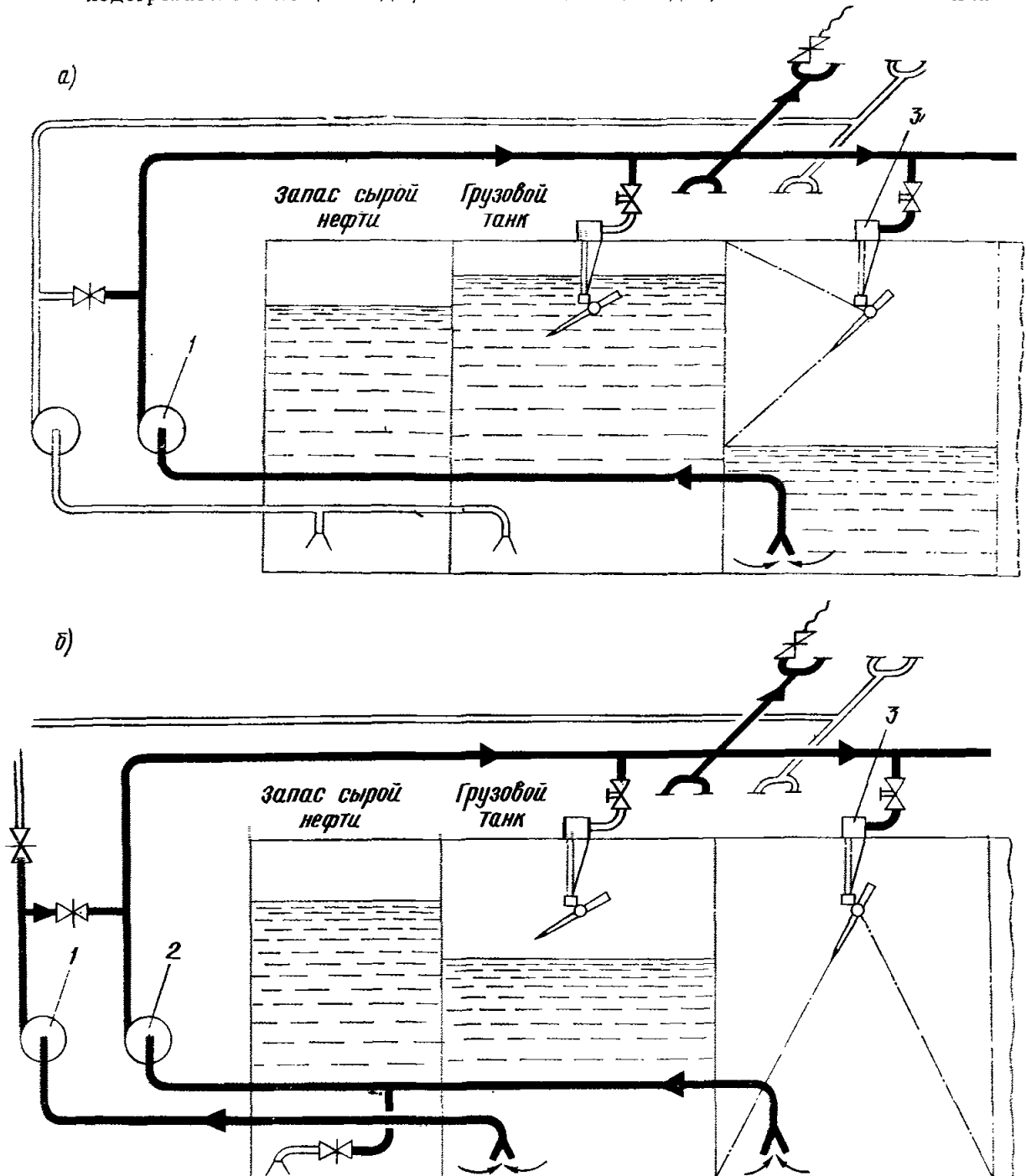
Рис. 5. Типовая схема мойки танков грузом сырой нефти двухэтапным способом: а — 1-й этап — мойка переборок; б — 2-й этап — мойка дна; 1 — грузовой насос, используемый для зачистки; 2 — зачистной насос; 3 — стационарная моечная машинка
