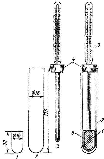
Рис. 9. Прибор для определения подвижности отложения:
