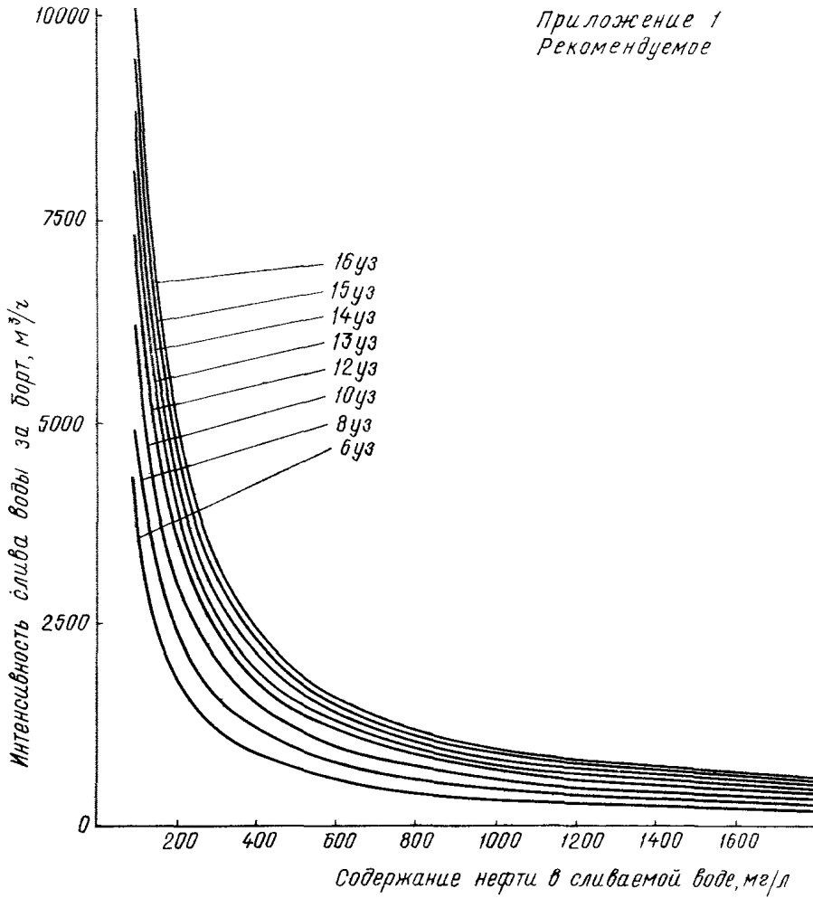
График для определения предельно допустимой интенсивности слива промывочной воды за борт (критерий 60 л/милю)
