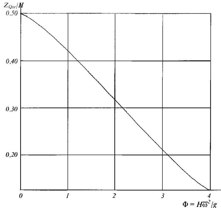
Рис. 3.1.4.13-2 Зависимость Z_{Qsr}/H от параметра \Phi = H\omega^2/g
