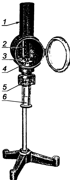
Рисунок 1 — Лампа для определения высоты некоптящего пламени
