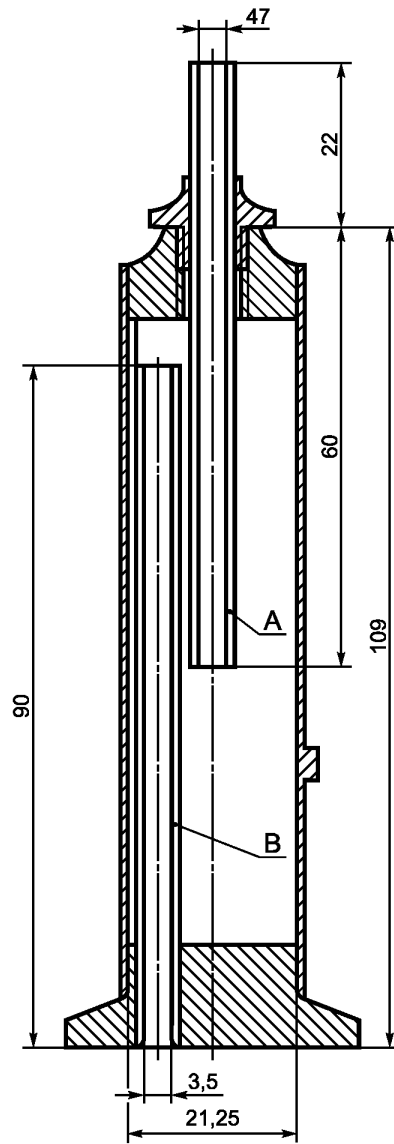
Рисунок А1.2 — Резервуар
