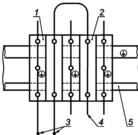
1 — клеммная колодка защитных проводников; 2 — клеммная колодка по ГОСТ Р 50030.7.1 ; 3 — испытательное напряжение; 4 — концы проводников; 5 — металлическое основание
