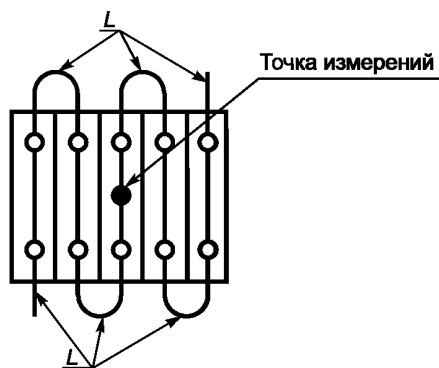
Рисунок 3 — Схема для испытания на превышение температуры (группа а)
