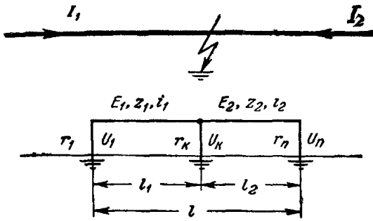
Рис. П7-5. Замыкание провода ВЛ на землю против одного из средних пунктов установки разрядников.
