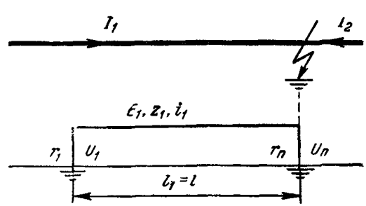
Рис. П7-6. Замыкание провода ВЛ на землю против конечного пункта установки разрядников.
