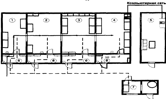
Рис. 1. Рекомендуемые схемы размещения помещений (рабочих зон) лаборатории, использующей МАНК с электроферретической и (или) гибридно-ферментативной детекцией продуктов амплификации (А и Б)
