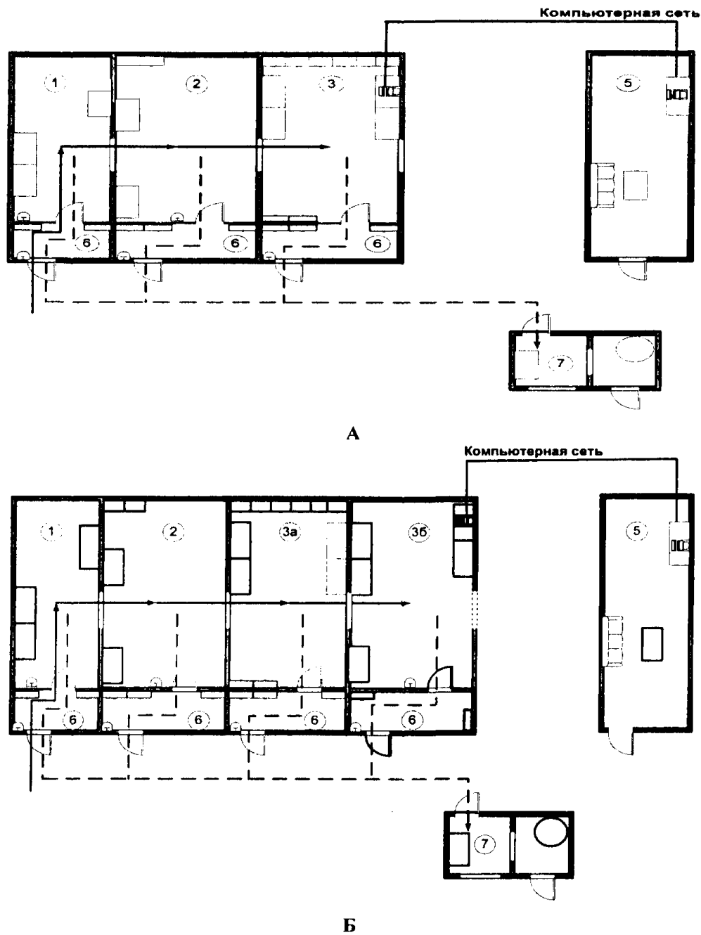
Рис. 2. Рекомендуемые схемы размещения помещений (рабочих зон) лаборатории, использующей МАНК с гибридно-флуоресцентным методом детекции продуктов амплификации (А и Б)
