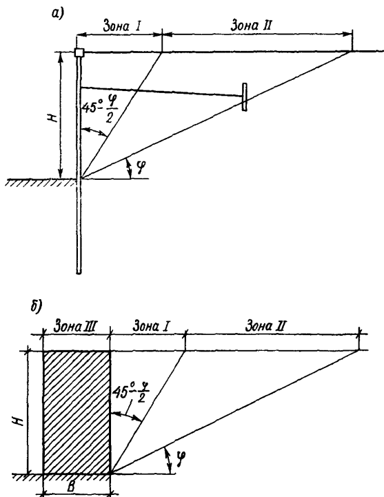
Рис. 1. Зоны загрузки опытных участков набережных: а – большерковкого типа; б – гравитационных
