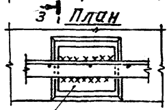
Закладная деталь (см. сер. 3.503-29)
