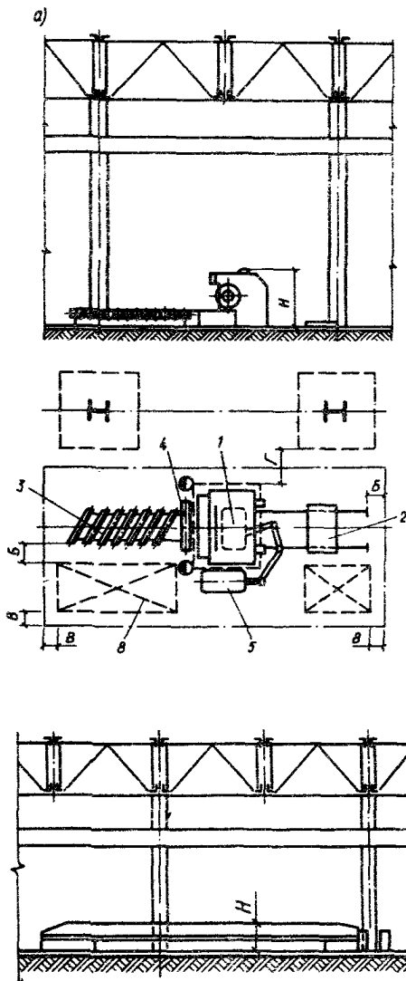
Рис.14. Размещение гильотинных ножиц при поперечной резке листа (а), при продольной резке листа (б)
