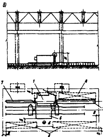
Рис.14. Размещение гильотинных ножиц при поперечной резке листа (а), при продольной резке листа (б)
