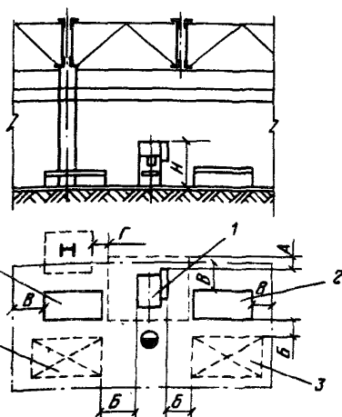
Рис. 9. Размещение прессы однокривошипного простого действия в продольном пролете 1 - пресс; 2 - стол к прессу; 3 - место складирования, A=400 мм, B=800 мм, B=500 мм, \Gamma=200 мм
