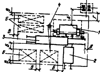
Рис. 6. Размещение сортогибочной машины в продольном пролете 1 - машина; 2 - козлок переставной; 3 - место складирования; А = 400 мм, В = 800 мм, В = 500 мм
