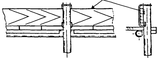
Крепление бортовой доски
