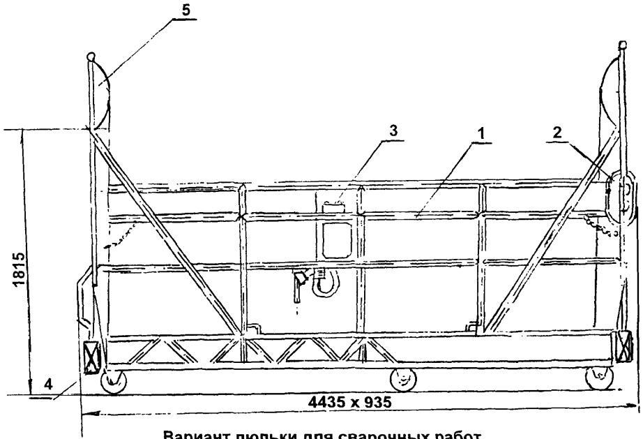
Вариант люльки для сварочных работ
