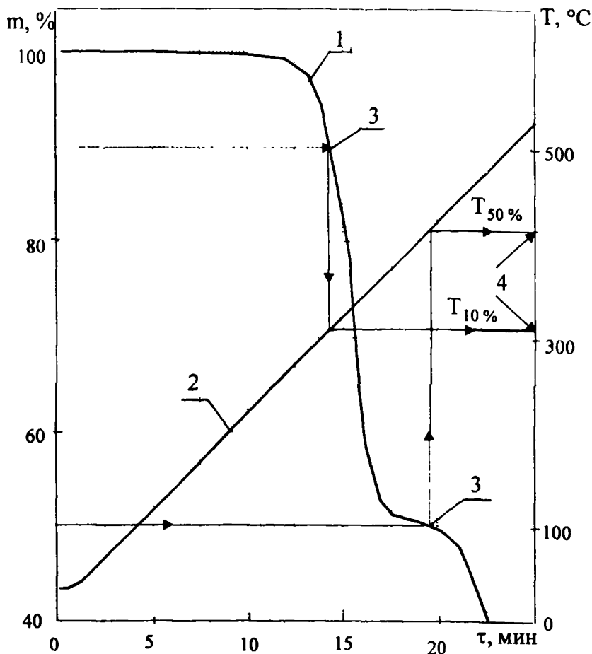
Рис. 2. Схема определения характерных температур при фиксированных значениях потери массы (в координатах потеря массы — время): 1 — ТГ-кривая (потеря массы); 2 — температура; 3 — характерные точки ТГ-кривой; 4 — температуры потери 10 и 50 % массы
