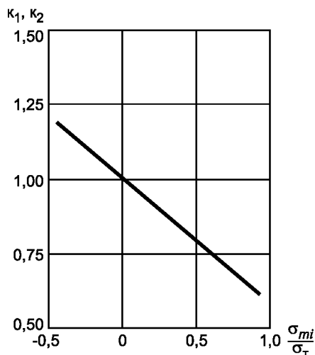
Рисунок А.1 — Диаграмма зависимости коэффициентов k_1, k_2 от значения относительной величины суммарных средних напряжений \frac{\sigma_{mi}}{\sigma_T}
