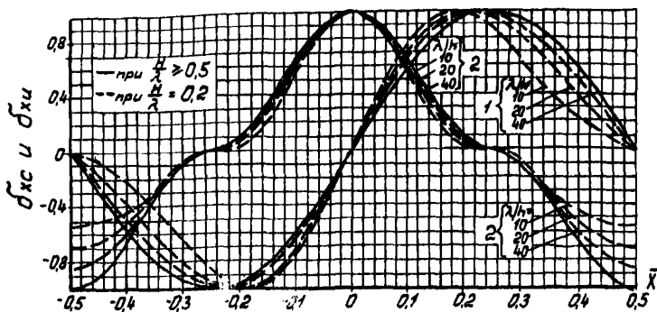
Рис.2. Графики значений коэффициентов сочетания инерционного \delta_{xс} (графики 1) и скоростного \delta_{xв} (графики 2) компонентов удельной горизонтальной нагрузки от волн
