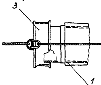
Рис. II. Схема плети:
