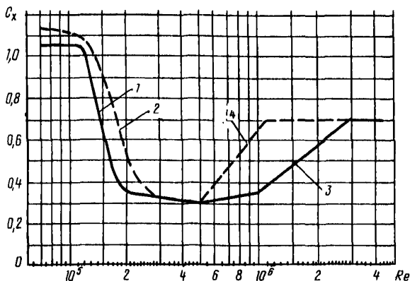
Рис.14. Значение коэффициента сопротивления трубы в поперечном потоке C_x :
