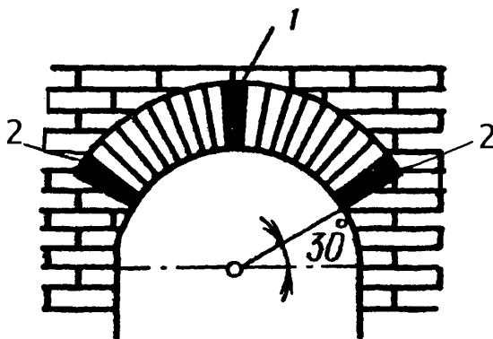
1 – замок; 2 – пяты
