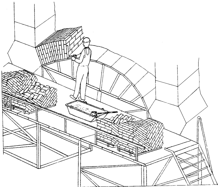
Рисунок 9 – Выверка кладки
