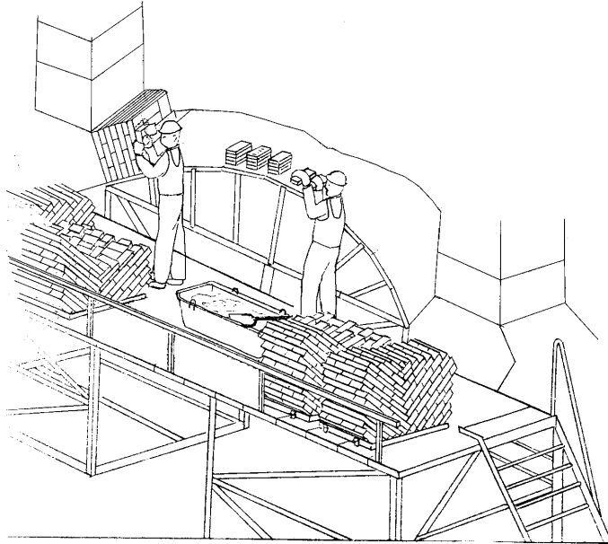
Рисунок 8 – Кладка арки (свода)
