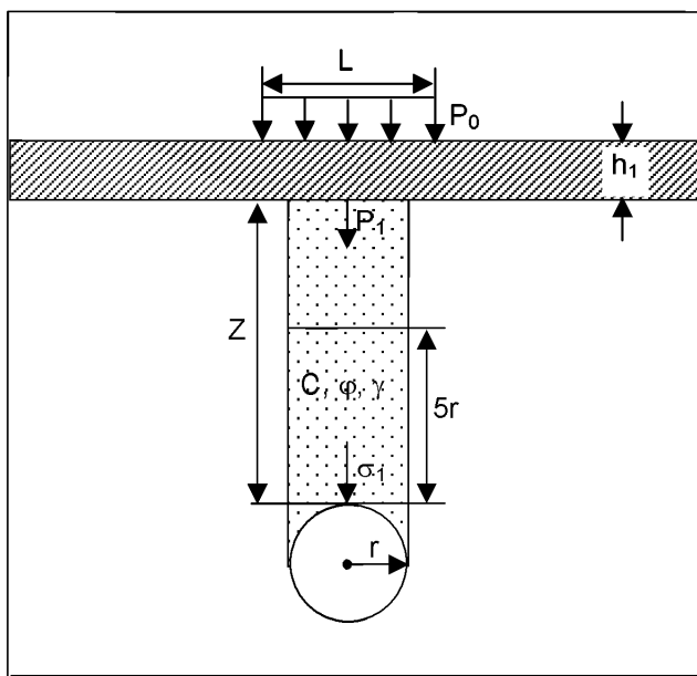
Рисунок 1 – Расчетная схема
