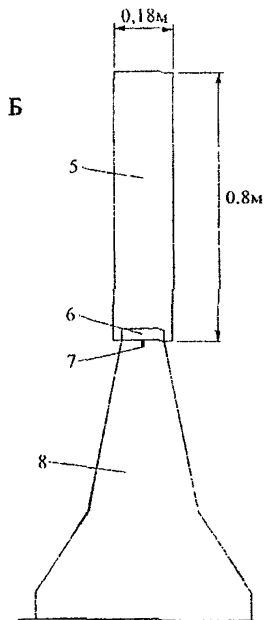
Рисунок 1 – Общий вид противоослепляющих экранов полимерных дорожных сетчатого типа (А) и пластинчатых (Б). Указанные цифровые значения – наиболее характерные
