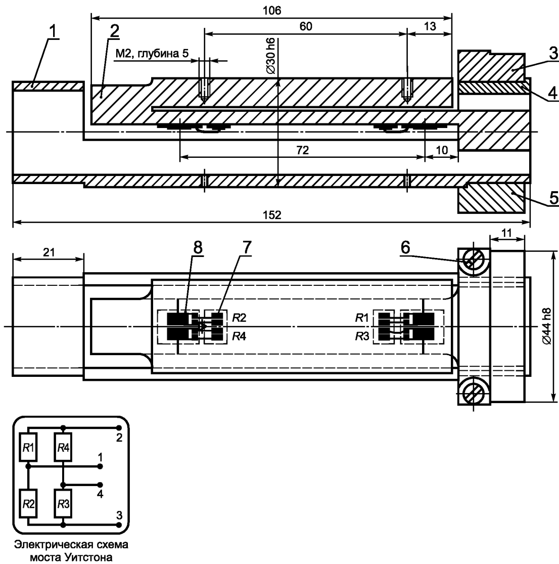
1 — рукоятка; 2 — измерительная пластина; 3 — стягивающее кольцо; 4 — площадка крепления; 5 — стягивающее кольцо; 6 — болт М2 × 16; 7 — паяный контакт; 8 — тензодатчик
