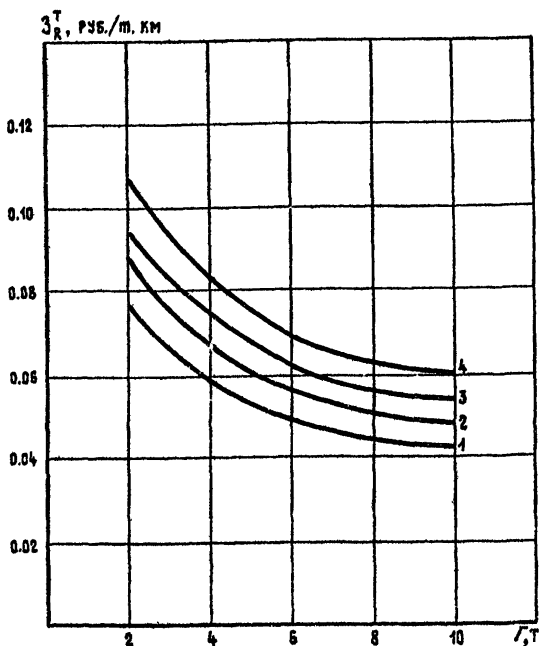
Рис. 2. График зависимости переменной составляющей приведенных затрат от грузоподъемности автотранспорта при перевозке топлива бортовыми автомобилями:
