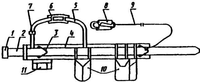
Рисунок 2 — Безлямочный пояс, тип Б
