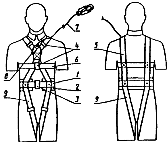
Рисунок 6 — Лямочный пояс, тип Е
