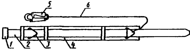
Рисунок 1 — Безлямочный пояс, тип А
