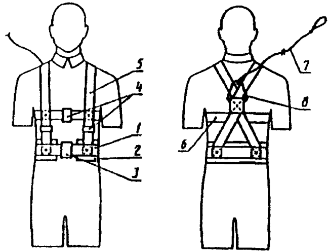
Рисунок 4 — Лямочный пояс, тип Г
