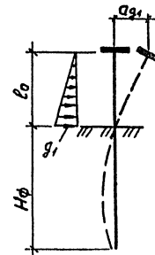
Расчетная схема №1
