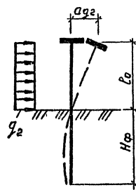
Расчетная схема №2
