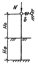
Расчетная схема для определения μ
