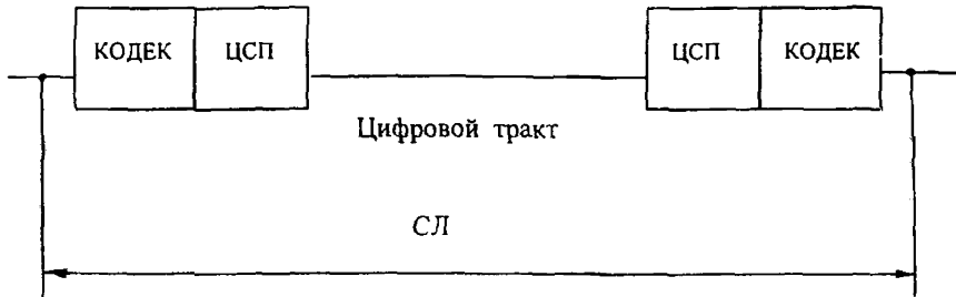
Рисунок 1 - Типовая структура цифровой СЛ
