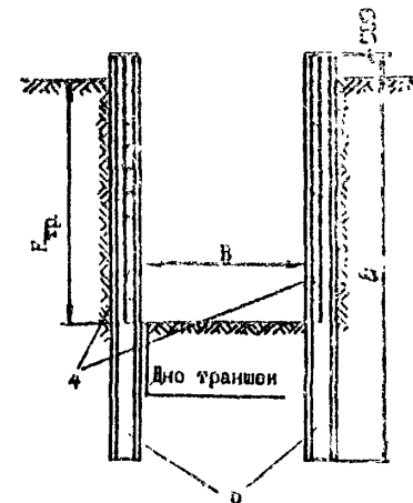
в) Консолями
