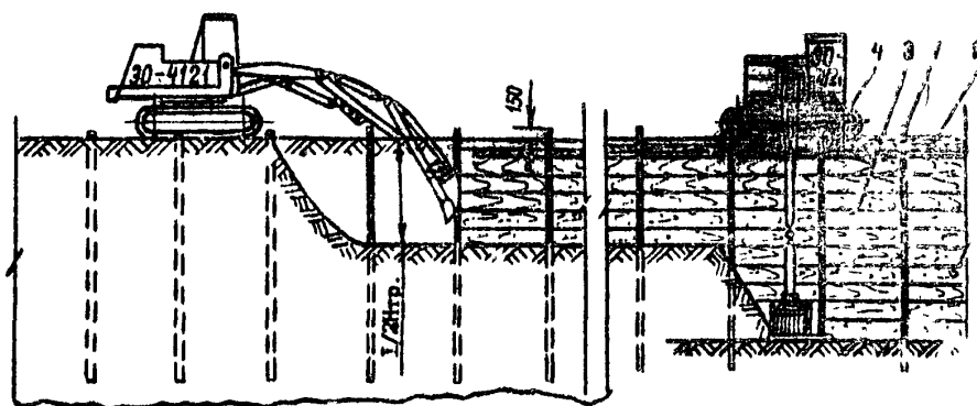
Разрез I-I
