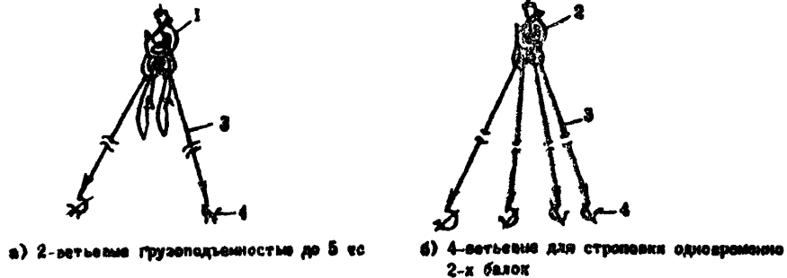
Схемы строповок
