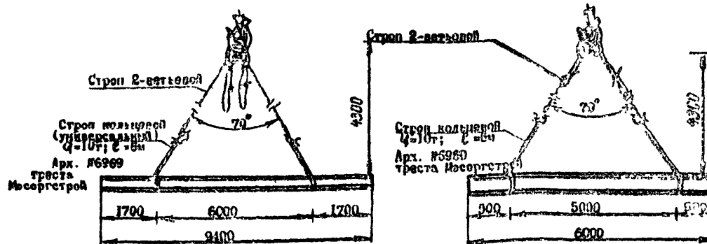
Схемы строповок
