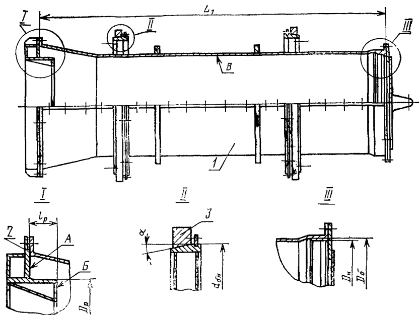
1 — корпус формы; 2 — раструбообразователь; 3 — бандаж
