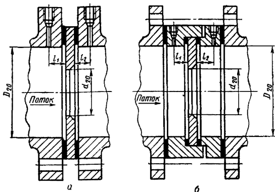
Рис. 4. Фланцевый способ отбора перепада давления для диафрагм
