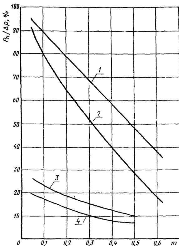
Рис. 8. Зависимость потери давления от типа и относительной площади сужающего устройства:
