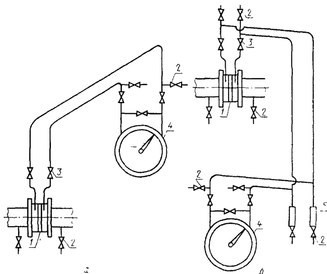
Рис. 9. Схемы соединительных линий при измерении расхода газа 1 — сужающее устройство; 2 — продувочный вентиль; 3 — вентиль; 4 — дифманометр; 5 — отстойный сосуд
