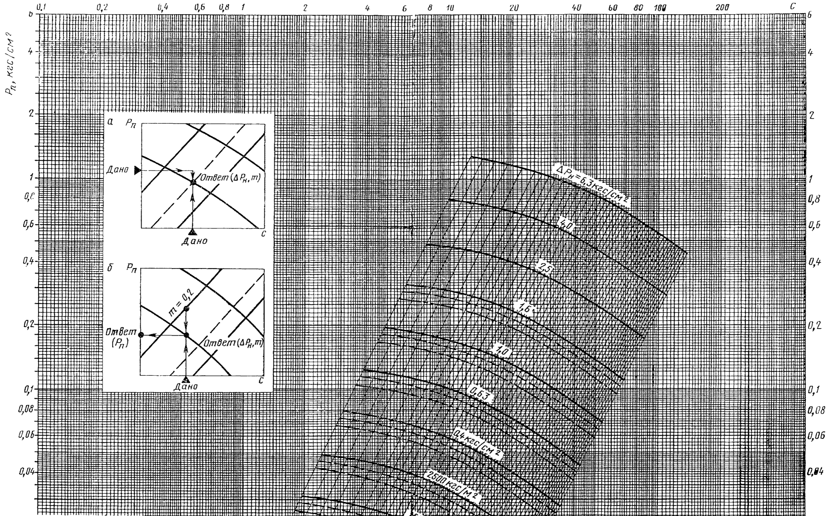
НОМОГРАММА ДЛЯ ОПРЕДЕЛЕНИЯ ПРЕДЕЛЬНОГО НОМИНАЛЬНОГО ПЕРЕПАДА ДАВЛЕНИЯ ДИФФЕРЕНЦИАЛЬНОГО ДИФФУЗИОННОГО И m -СОПЕЛ ВЕНТУРИ
