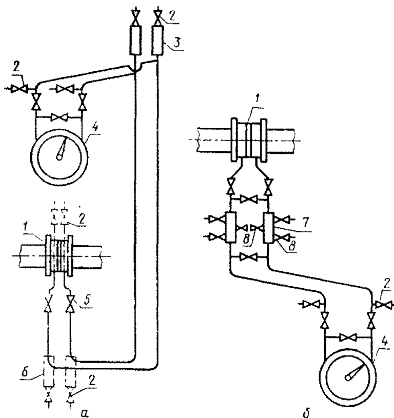
Рис. 12. Схемы соединительных линий при измерении расхода жидкости: 1 — сужающее устройство; 2 — продувочный вентиль; 3 — газосборник; 4 — дифманометр, 5 — вентиль, 6 — отстойный сосуд; 7 — разделяющий сосуд; 8 — контрольный вентиль
