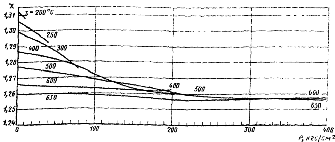
ПОКАЗАТЕЛЬ АДИАБАТЫ ПЕРЕГРЕТОГО ВОДЯНОГО ПАРА
