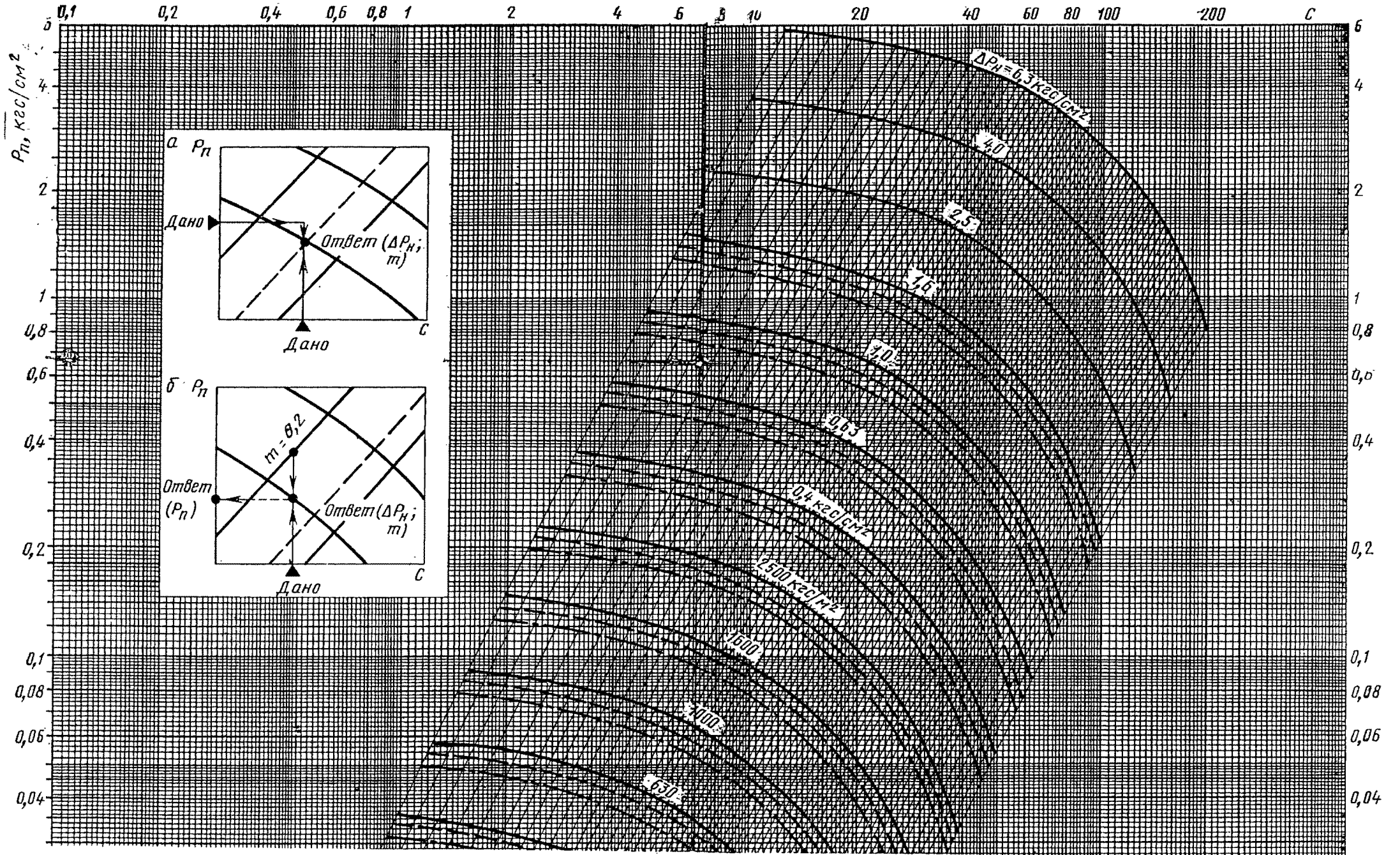
НОМОГРАММА ДЛЯ ОПРЕДЕЛЕНИЯ ПРЕДЕЛЬНОГО НОМИНАЛЬНОГО ПЕРЕПАДА ДАВЛЕНИЯ ДИФФАНОМЕТРА И m -СОПЕЛ
