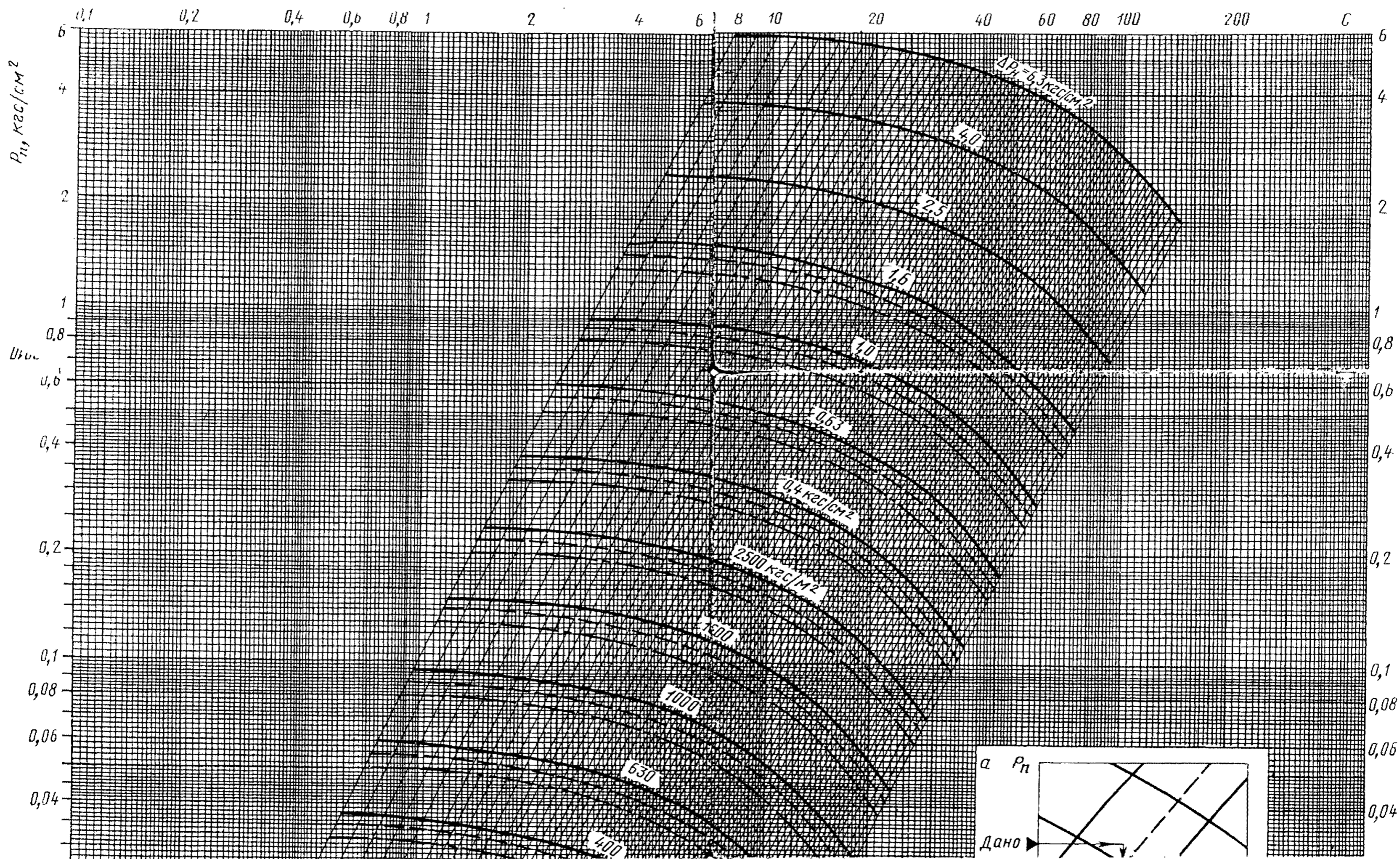
НОМОГРАММА ДЛЯ ОПРЕДЕЛЕНИЯ ПРЕДЕЛЬНОГО НОМИНАЛЬНОГО ПЕРЕПАДА ДАВЛЕНИЯ ДИФФЕРЕНЦИАЛЬНОГО ДИФФРАГМА И m -ДИАФРАГМА
