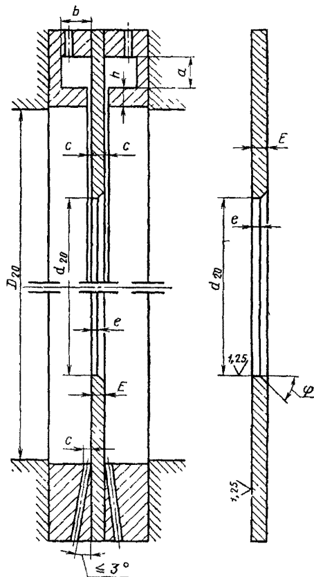
Рис. 3. Основные геометрические размеры стандартных диафрагм
