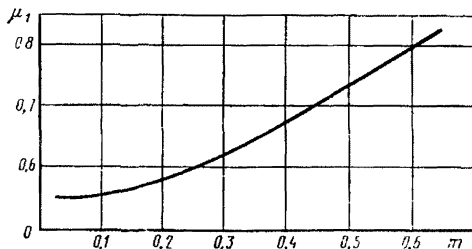
Рис. 1. Коэффициент сужения струи
