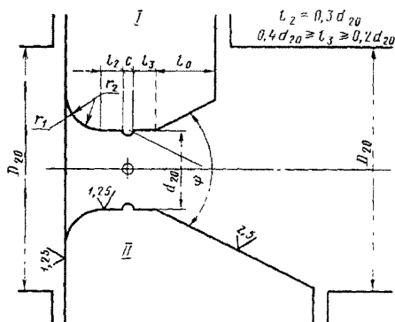
Рис 6 Основные геометрические параметры сопел Вентури:
