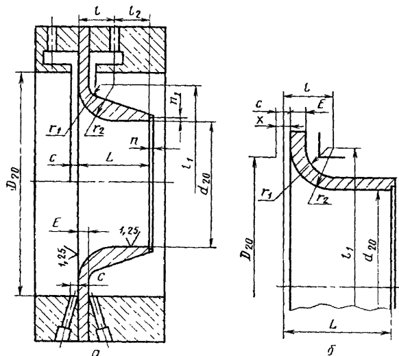
Рис 5. Основные геометрические параметры сопел: а — для m \leq 0,444 ; б — для m > 0,444
