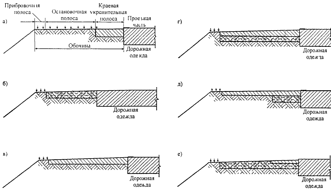
Рис. 2. Конструктивные решения по укреплению обочин
