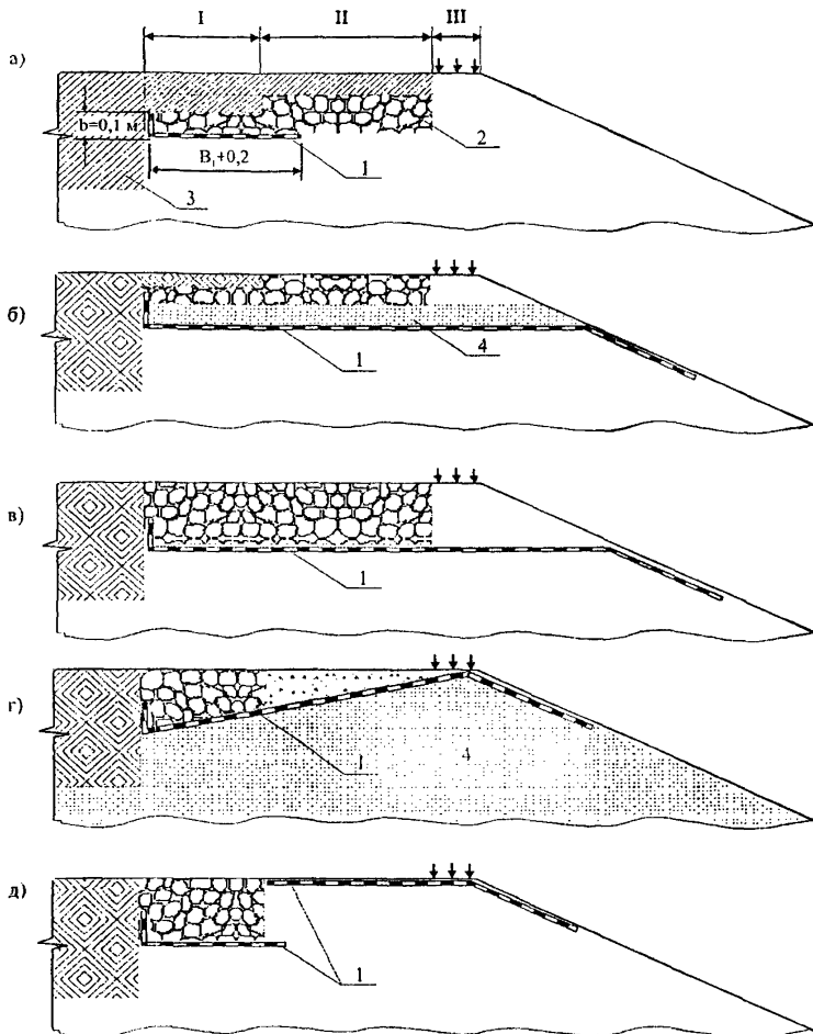
Рис. 3. Основные варианты применения ГМ при укреплении обочины:
