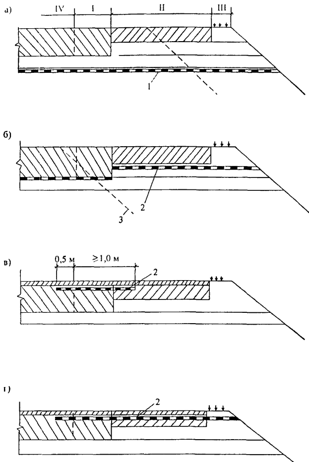
Рис. 4. Усиление конструкций укрепления обочины при уширении земляного полотна и дорожной одежды: I – краевая укрепительная полоса; II – остановочная полоса; III – прировочная полоса; IV – полоса уширения проезжей части; 1 – защитно-дренирующая полоса из ГМ; 2 – армирующая прослойка из ГМ; 3 – граница уширяемой части насыпи
