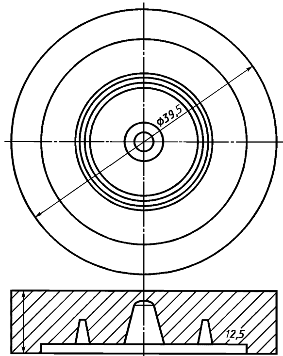
Рисунок 4 — Форма для изготовления образцов
