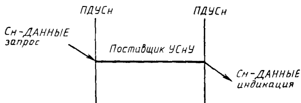
Рисунок 6 — Последовательность примитивов услуги Сн-ДААННЫЕ
