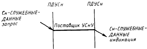
Рисунок 8 — Последовательность примитивов услуги Сл-СЛУЖЕБНЫЕ-ДААННЫЕ
