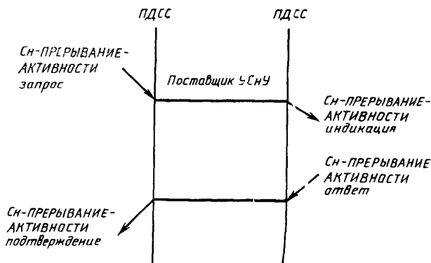
Рисунок 20 — Последовательность примитивов услуги СН-ПРЕРЫВАНИЕ-АКТИВНОСТИ
