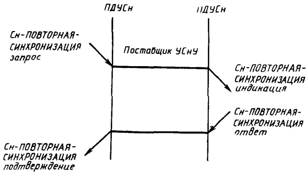
Рисунок 15 — Последовательность примитивов услуги Сн-ПОВТОРНАЯ-СИНХРОНИЗАЦИЯ
