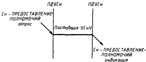
Рисунок 10 — Последовательность примитивов услуги Сн-ПРЕДОСТАВЛЕНИЕ-ПОЛНОМОЧИЙ
