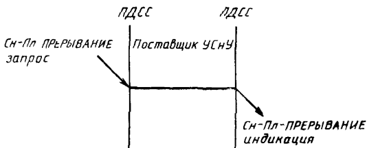
Рисунок 24 — Последовательность примитивов услуги Сн Пл ПРЕРЫВАНИЕ
