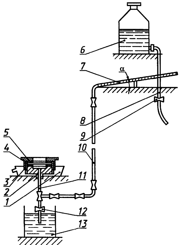
1 — ванна; 2 — полная камера; 3 — крышка; 4 — резиновая уплотняющая прокладка; 5 — металлическая прокладка; 6 — сосуд с тубусом для воды; 7 — стеклянная градуированная трубка; 8, 11 — резиновые трубки; 9, 12 — зажимы на трубках; 10 — стеклянная трубка; 13 — бачок для слива воды
