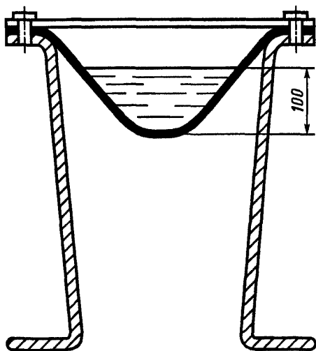
Рисунок 4 — Приспособление для определения водонепроницаемости методом кошеля
