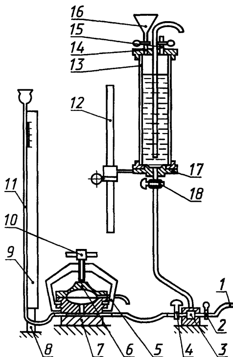
1 — спускная трубка; 2—4 — краны; 5 — трубица; 6 — крышка; 7 — основание; 8 — стойка; 9 — шкала давления; 10 — винт; 11 — трубка; 12 — штатив; 13 — стеклянный цилиндр; 14 и 15 — краны; 16 — воронка; 17 — держатель штатива; 18 — кран
