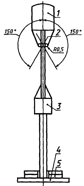
1 — верхний подвижный зажим; 2 — губки подвижного зажима; 3 — нижний подвижный зажим; 4 — площадка для грузов; 5 — грузы
