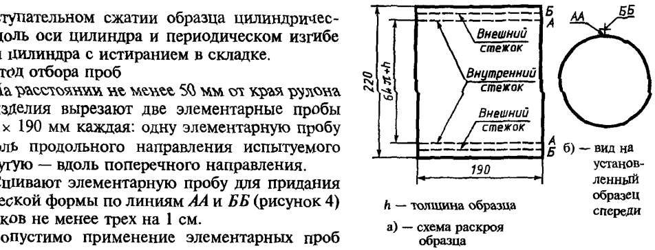
Рисунок 4 — Подготовка образца при испытании методом истирания в складке (метод В)
