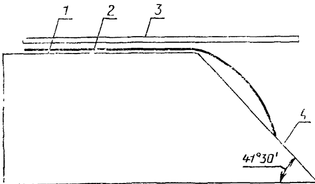
1 — горизонтальная платформа, 2 — элементарная проба ткани, 3 — ползун линейки, 4 — наклонная платформа
